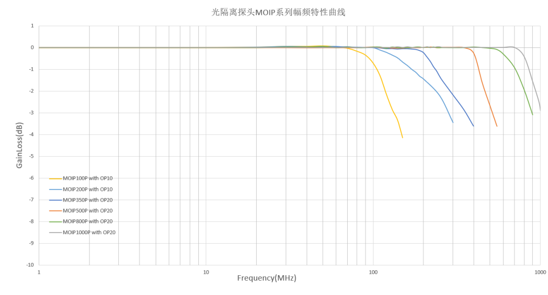
上图展示不同型号光隔离探头的幅频特性
