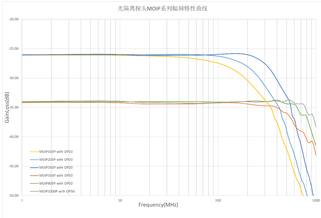
上图展示不同型号光隔离探头的幅频特性
