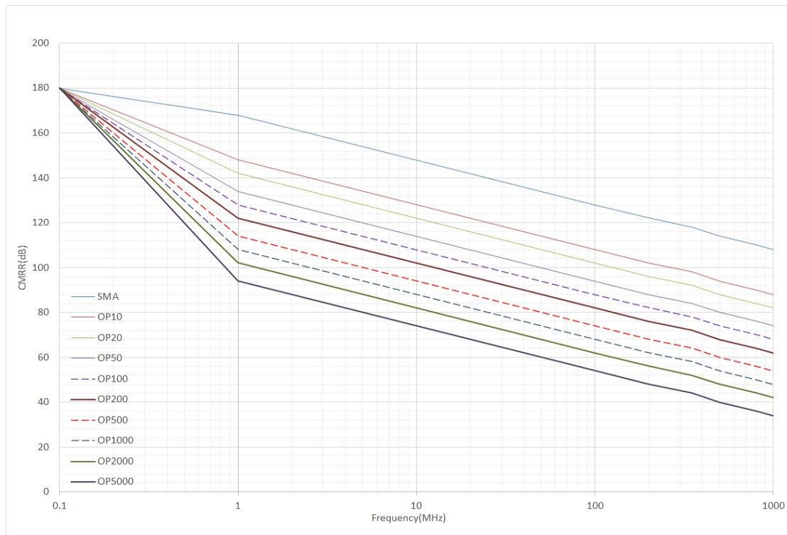
上图展示不同型号衰减器（0dB）在各个频率下的共模抑制能力。
