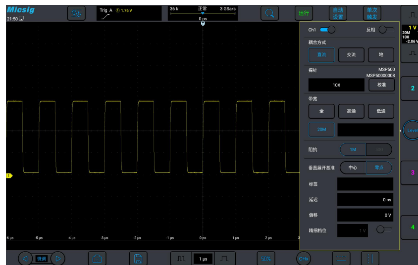
图5-11 20M带宽
