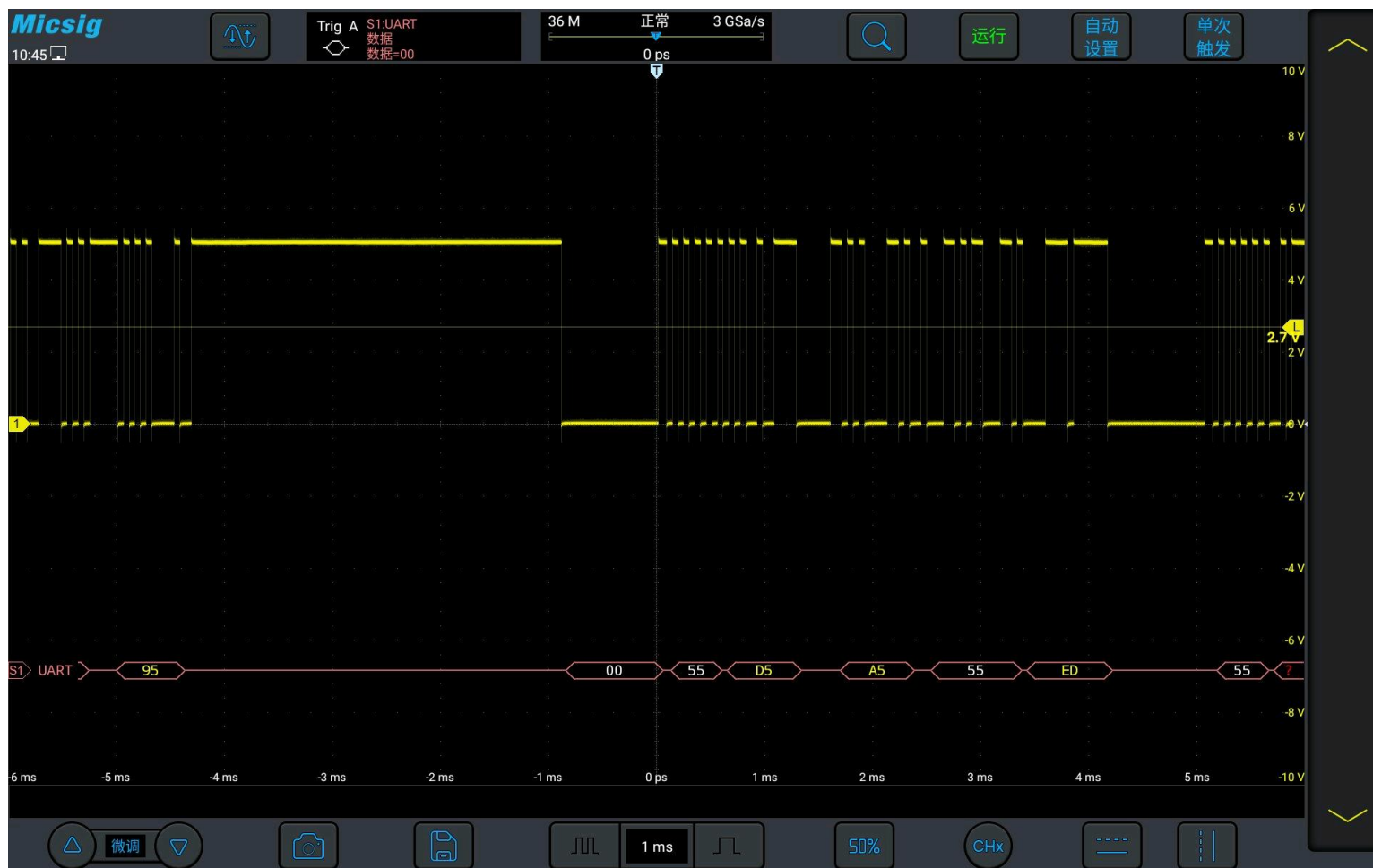
图 12-7 UART 解码阈值电平调节
