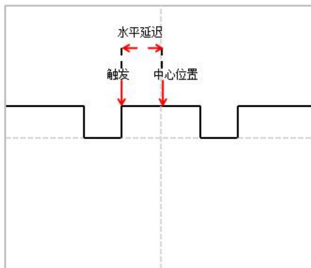
图 6-7 水平延迟
