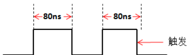
图6-14 触发时间 T < 80\text{ns}
