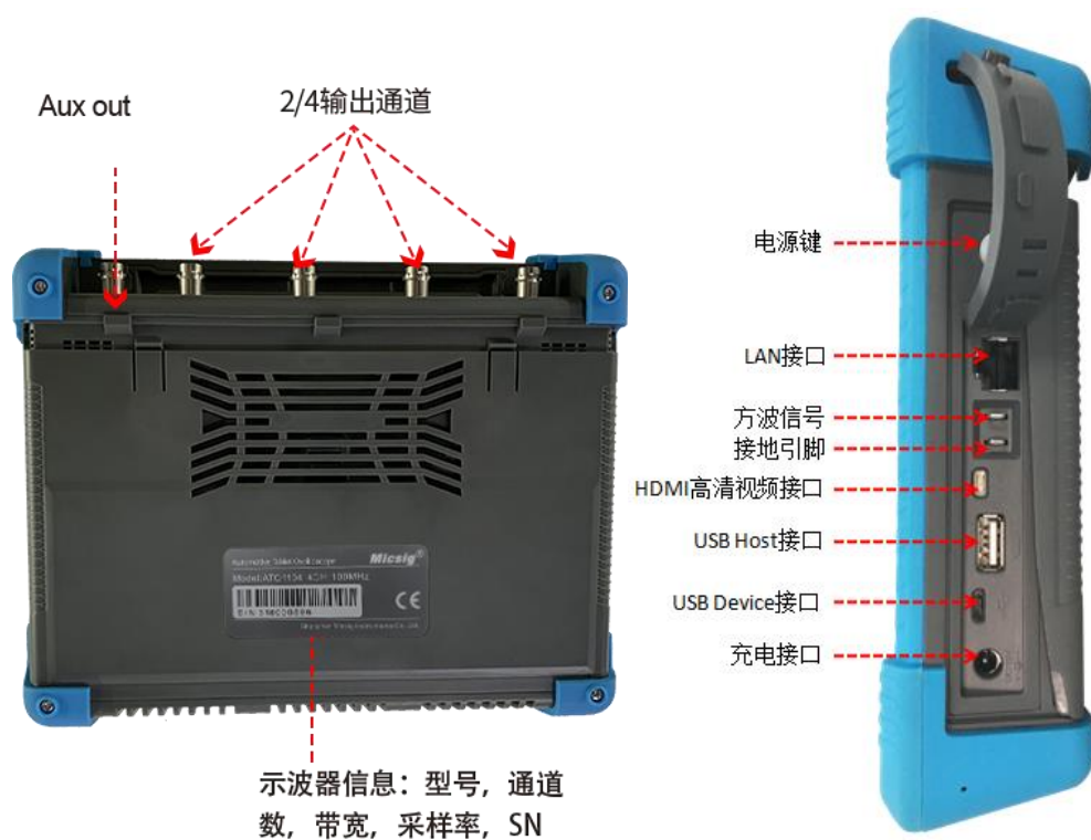
图2-2 背面板&侧面板
