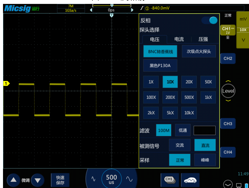
图5-13 反相后
