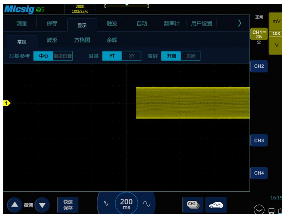
图4-6 滚屏模式
