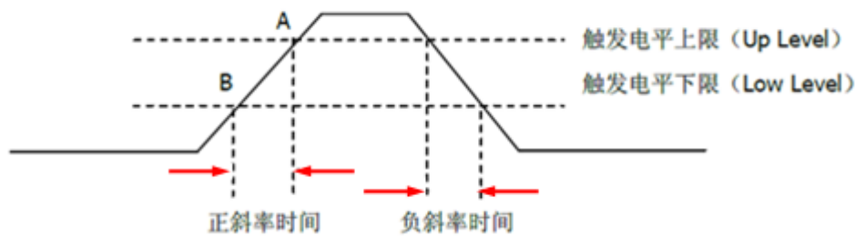
图6-24 正斜率时间/负斜率时间
