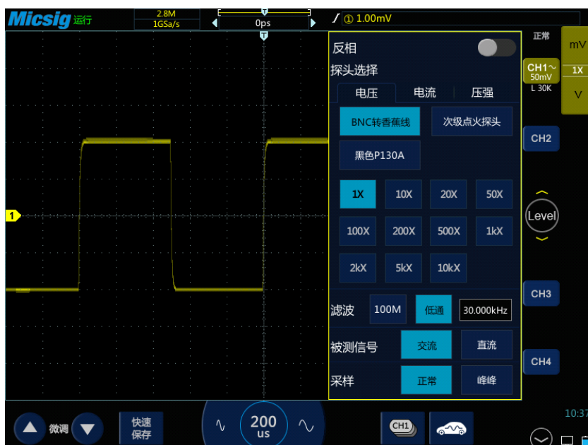
图5-11 低通
