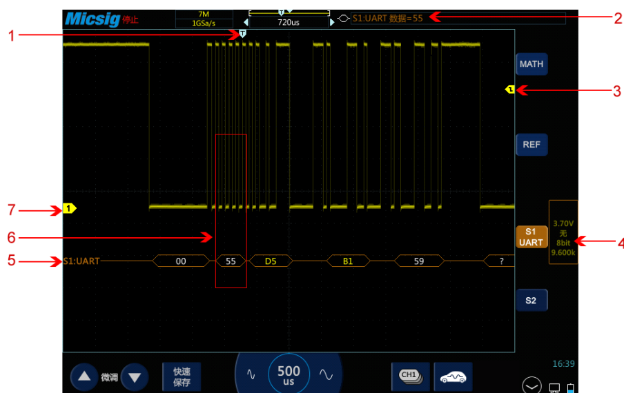
图14-8 UART 文本界面
