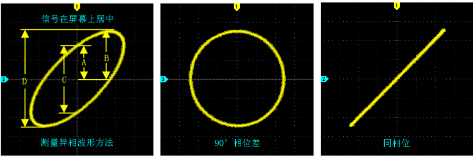
图4-8 XY 时基模式信号，在显示屏上居中
