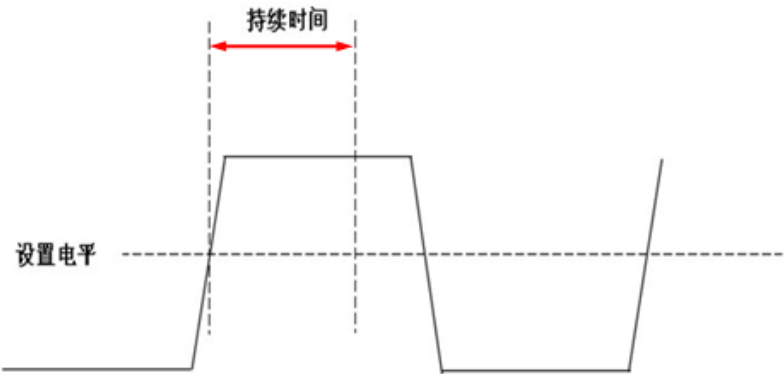
图6-26 超时触发示意图
