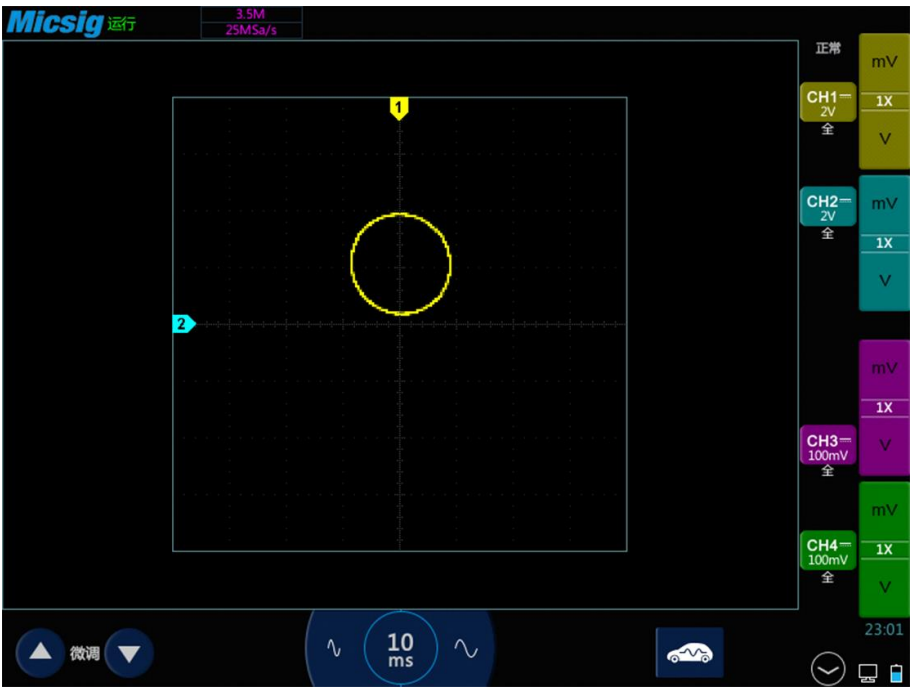
图4-7 XY 模式
