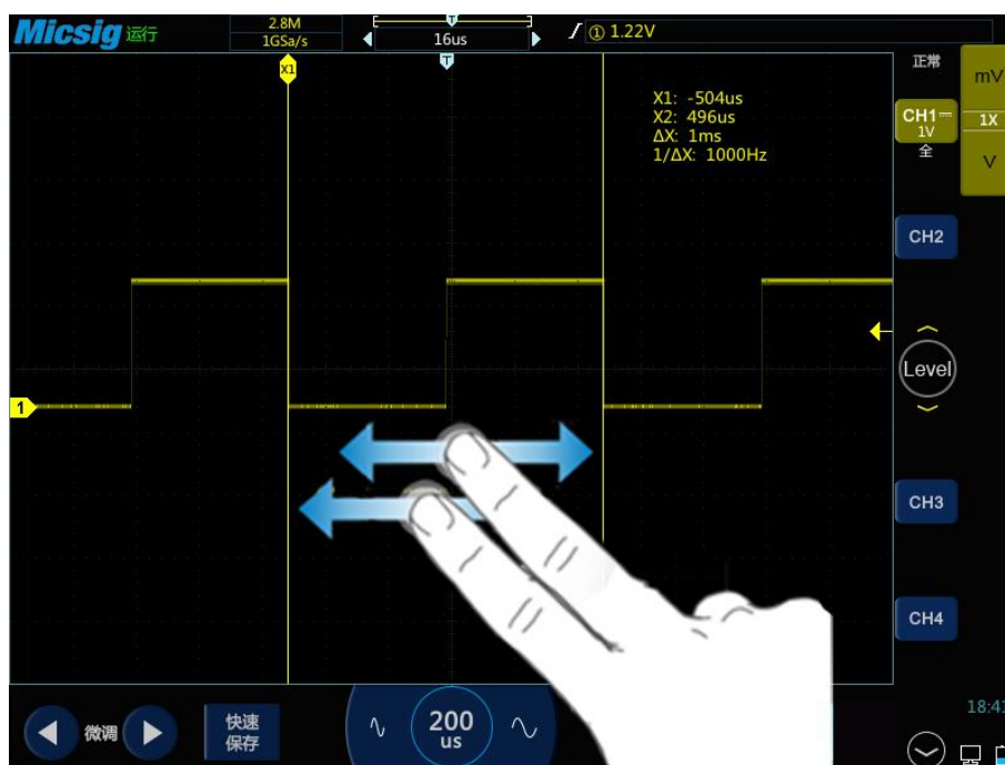
图7-9 光标测量脉冲宽度
