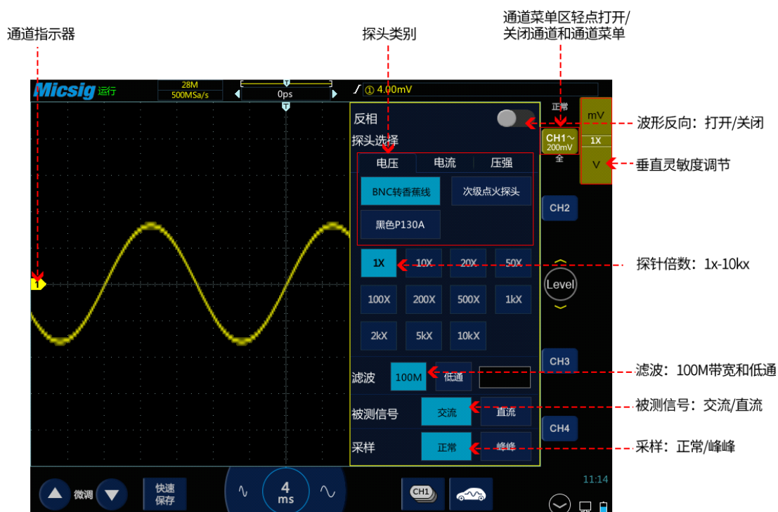
图5-1 通道菜单显示界面
