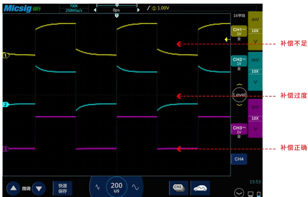
图2-13 探头补偿
