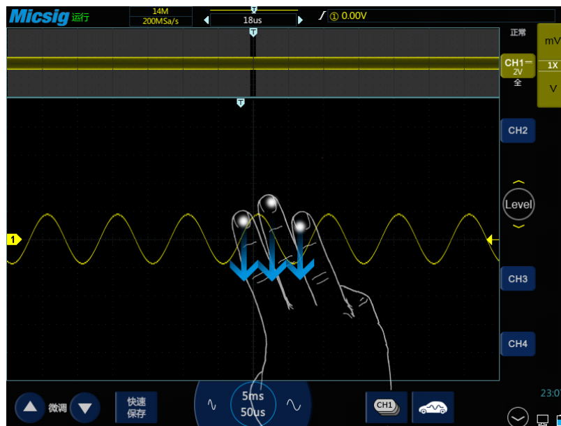
图4-11 三指下滑打开 Zoom 功能
