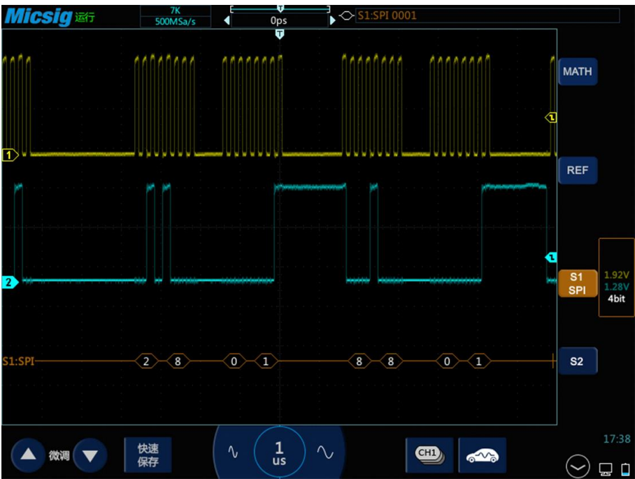
图14-19 SPI 图形界面
