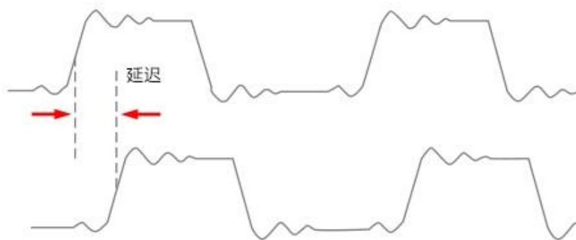
图7-4 延迟测量示意图
