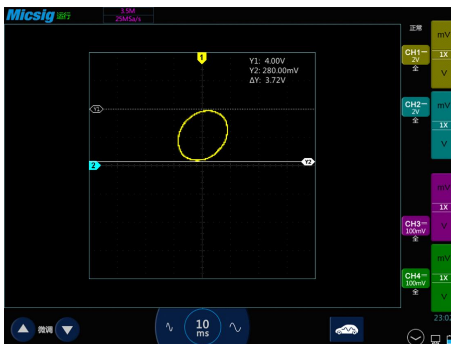
图7-10 XY 模式中，光标测量
