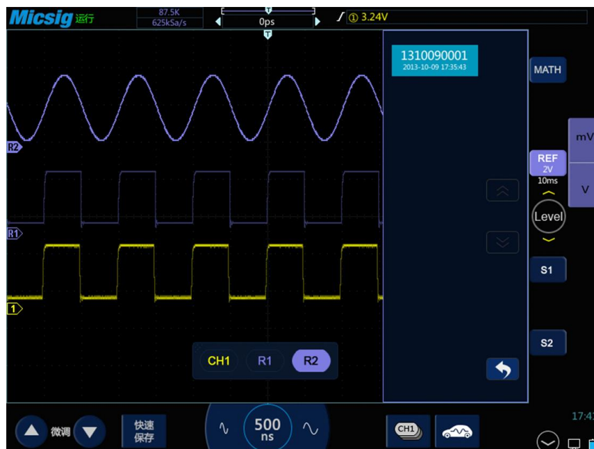
图9-7 恢复参考波形
