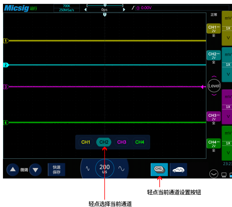
图5-5 使用当前通道选择按钮
