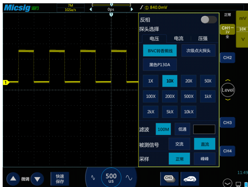
图5-12 反相前
