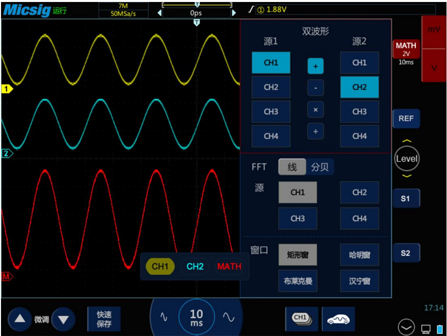
图9-3 通道 1 加通道 2 数学运算示图
