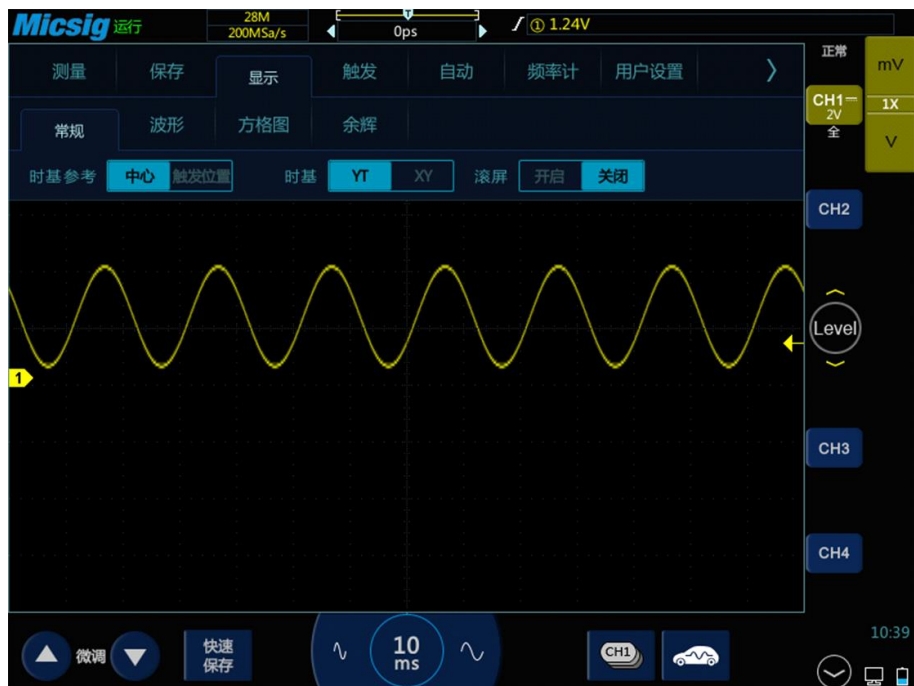
图10-1 显示设置和功能键
