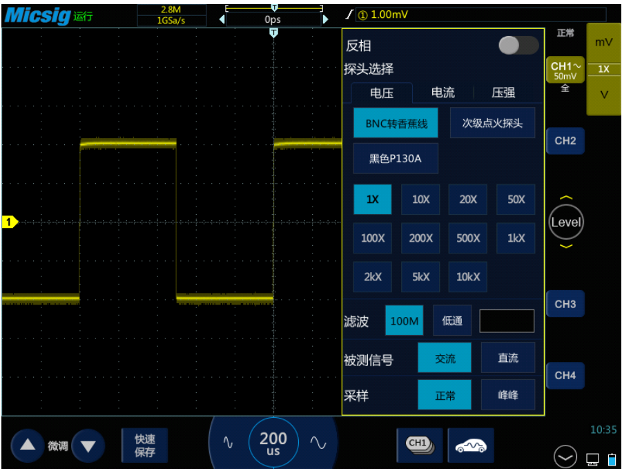
图5-9 交流
