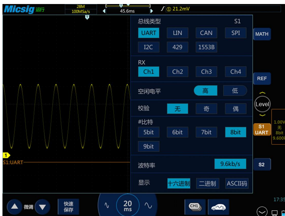
图14-4 UART 总线配置菜单
