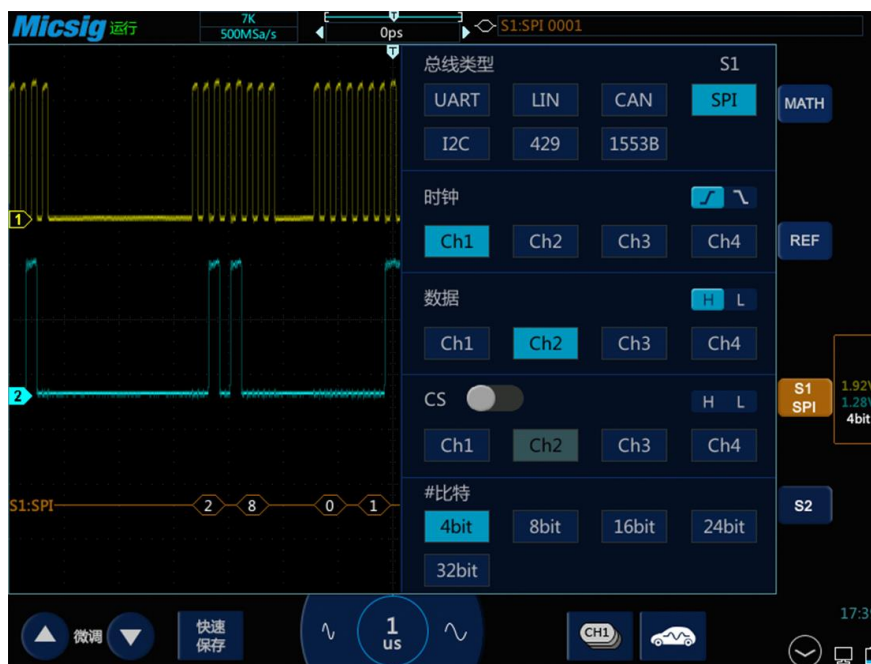
图14-17 SPI 总线配置菜单
