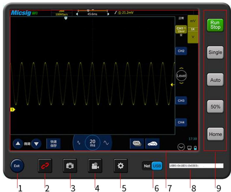
图13-2 上位机界面
