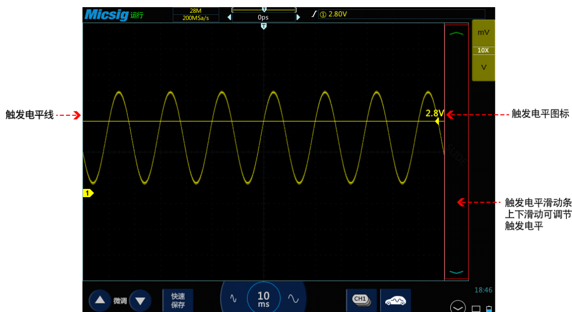
图6-8 触发电平
