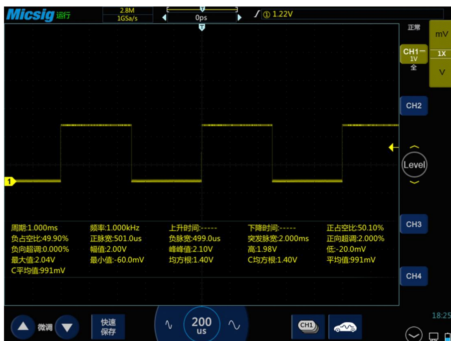
图7-3 全部测量
