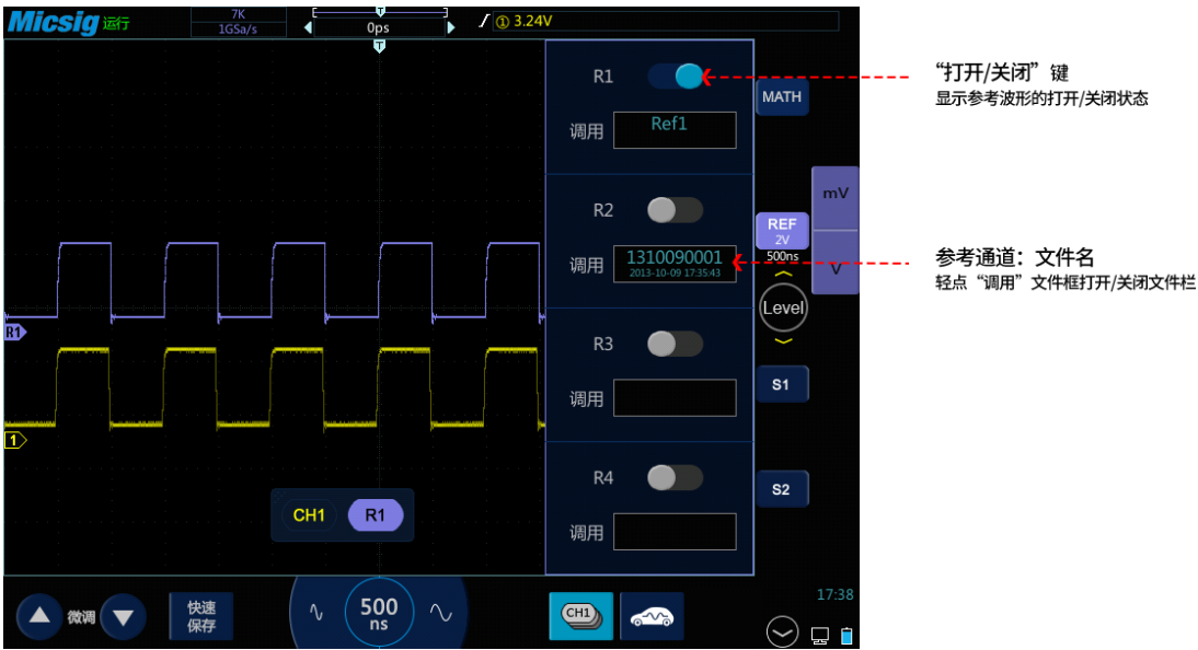
图9-6 参考通道菜单
