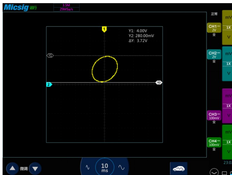
图4-9 相差测量和使用光标
