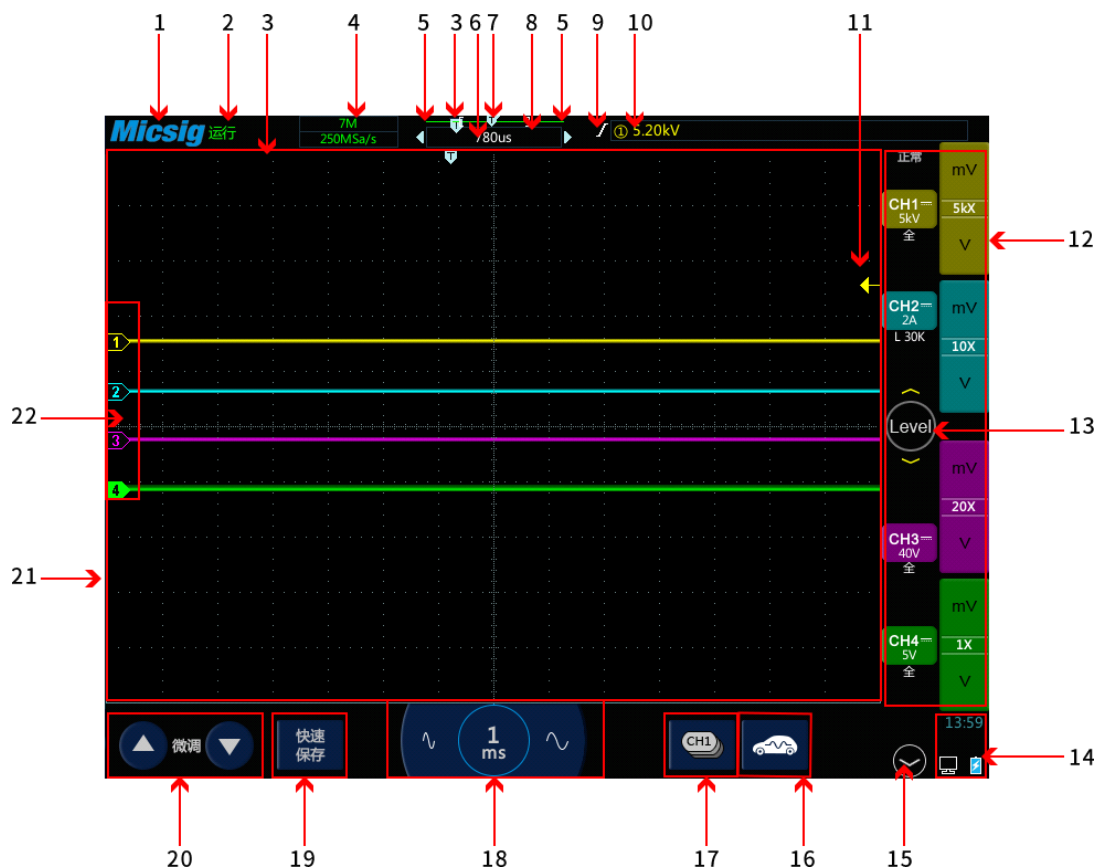
图2-4 示波器界面显示
