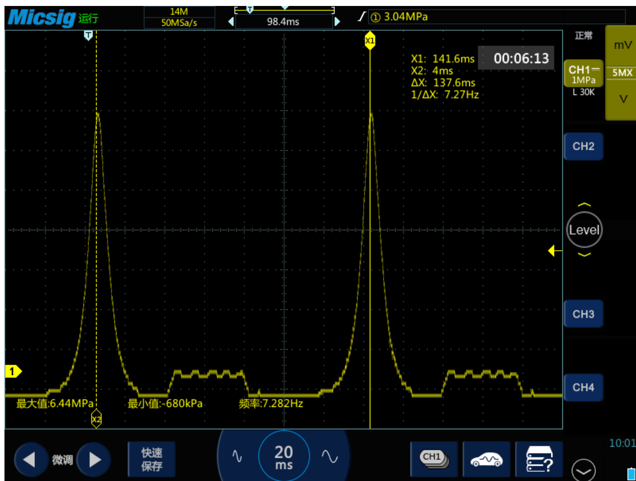
图3-62 气缸内部压力实测
