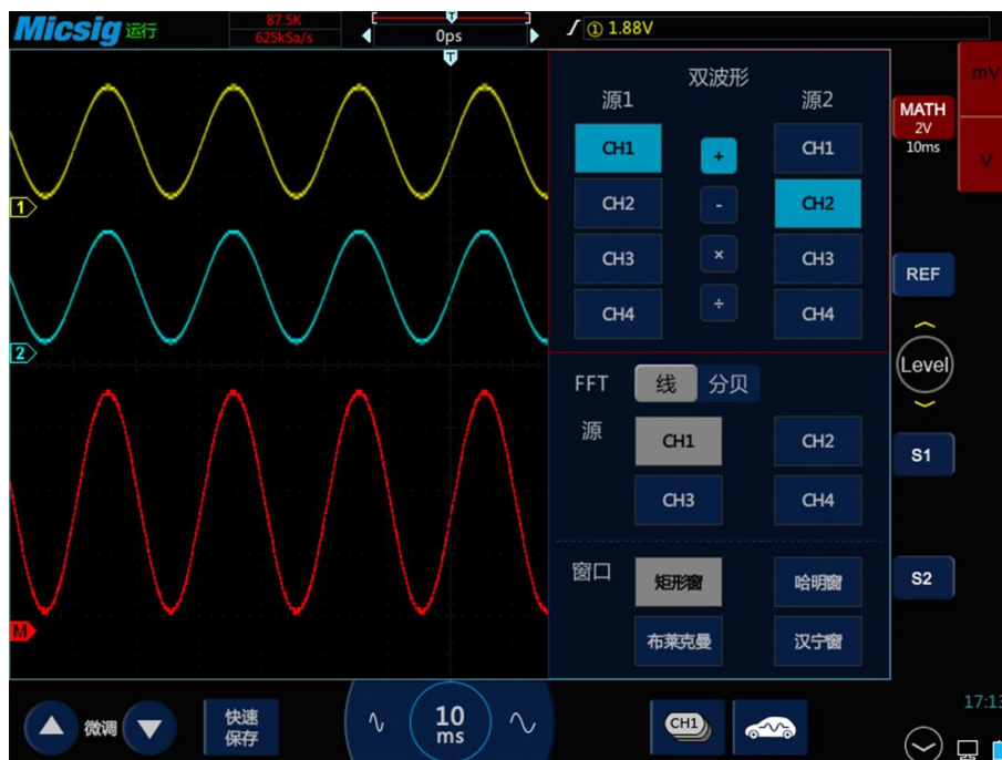
图9-1 数学通道
