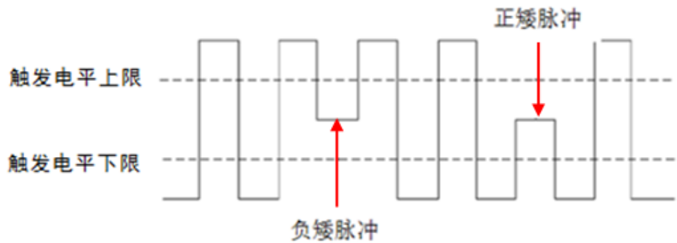
图6-22 欠幅触发
