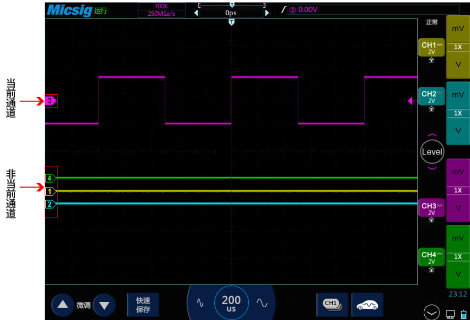
图5-2 当前通与非当前通道
