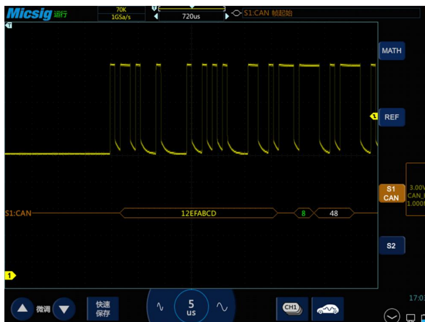
图14-15 CAN 图形界面
