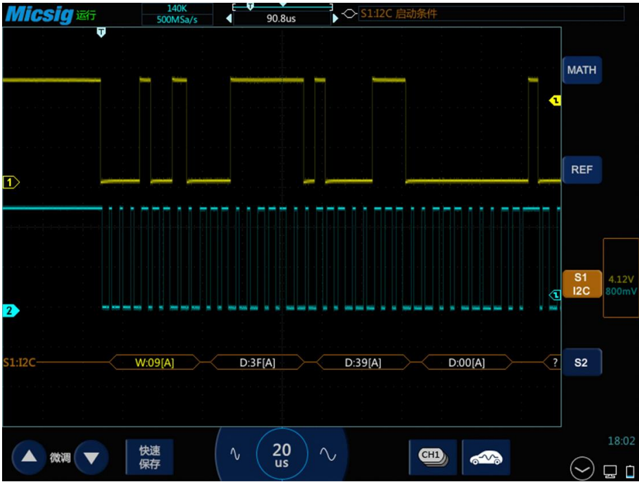
图14-23 I2C 图形界面
