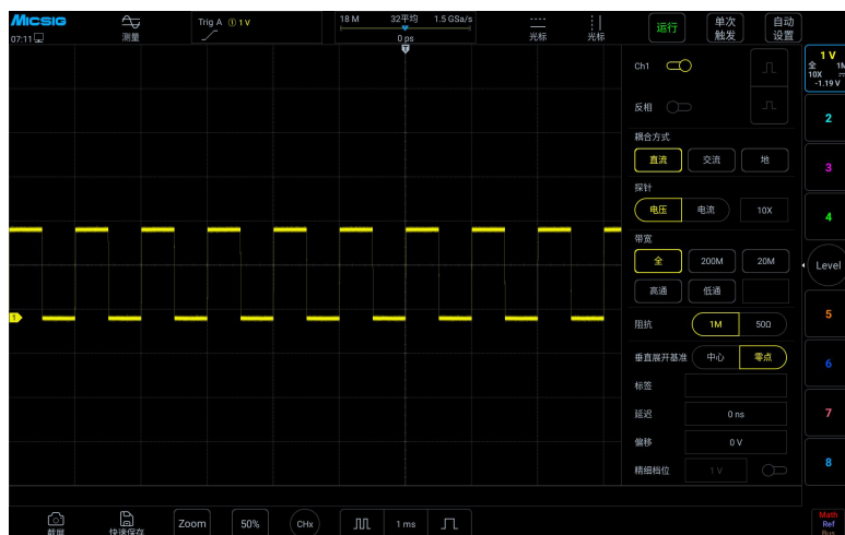
图5-10 全带宽
