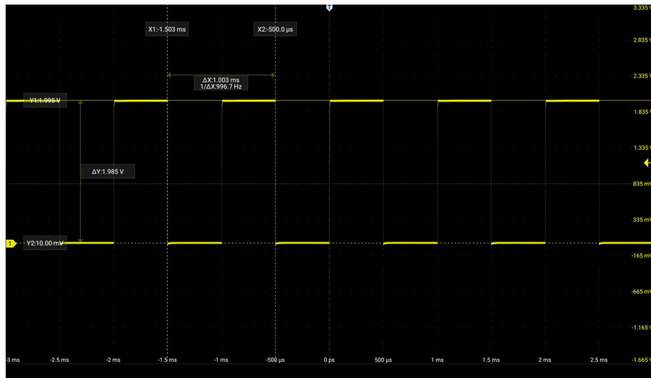
图 7-16 光标测量
