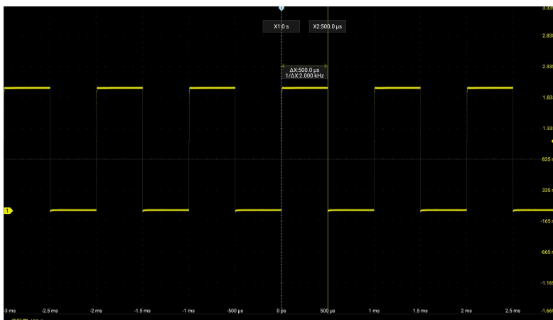
图 7-18 光标测量脉冲宽度
