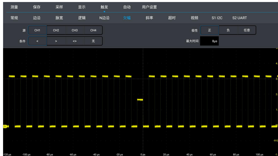
图 6-25 欠幅触发设置菜单
