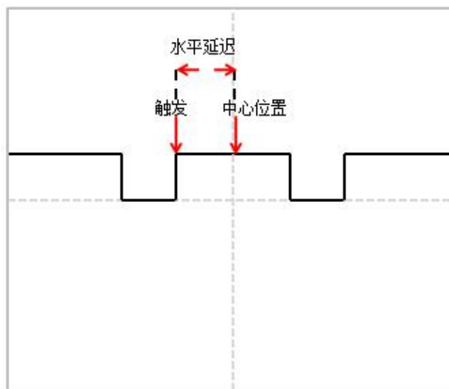
图 6-7 水平延迟
