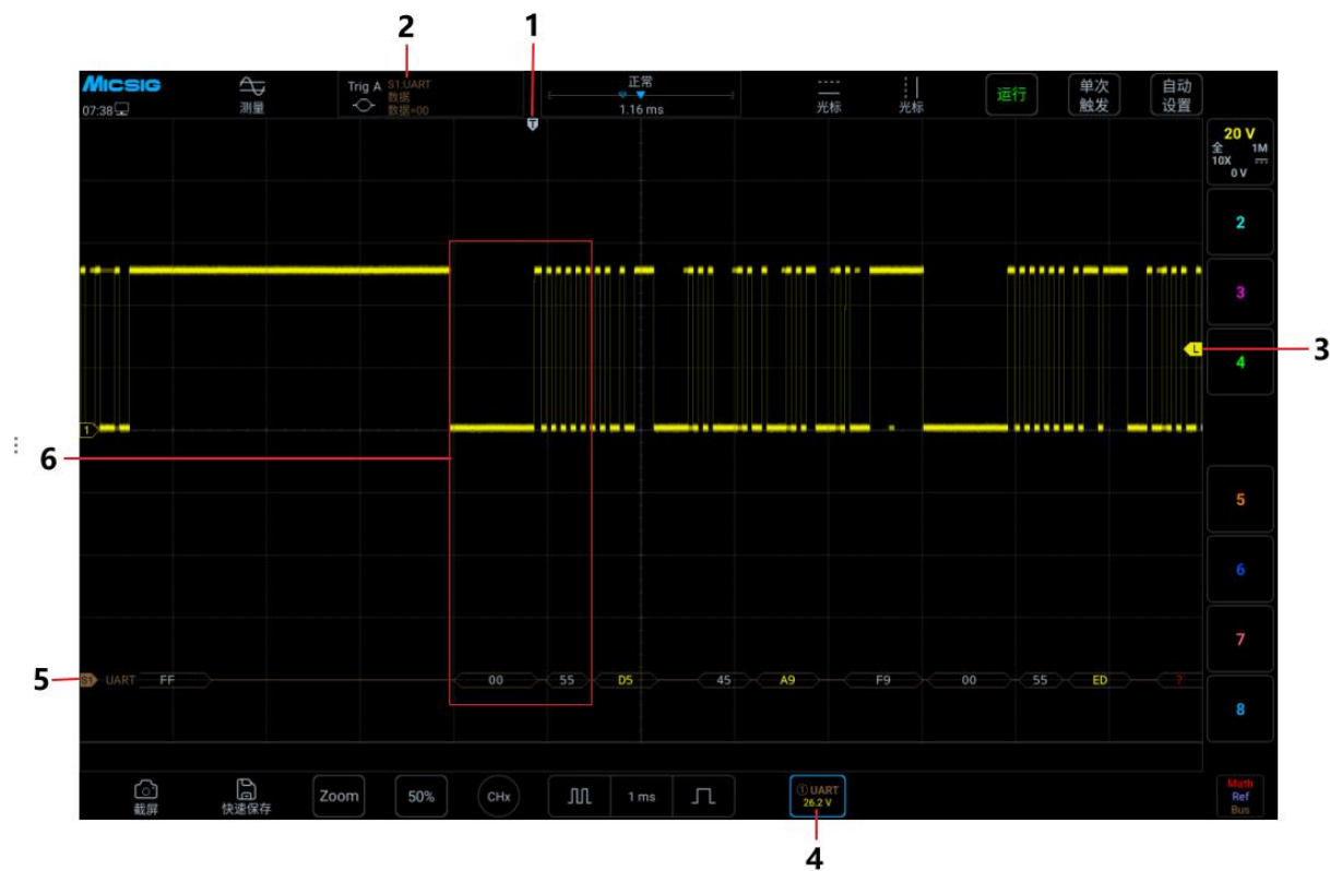
图 12-8 UART 图形界面
