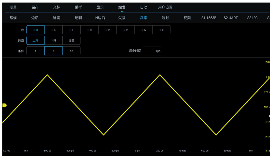
图 6-27 斜率触发设置菜单
