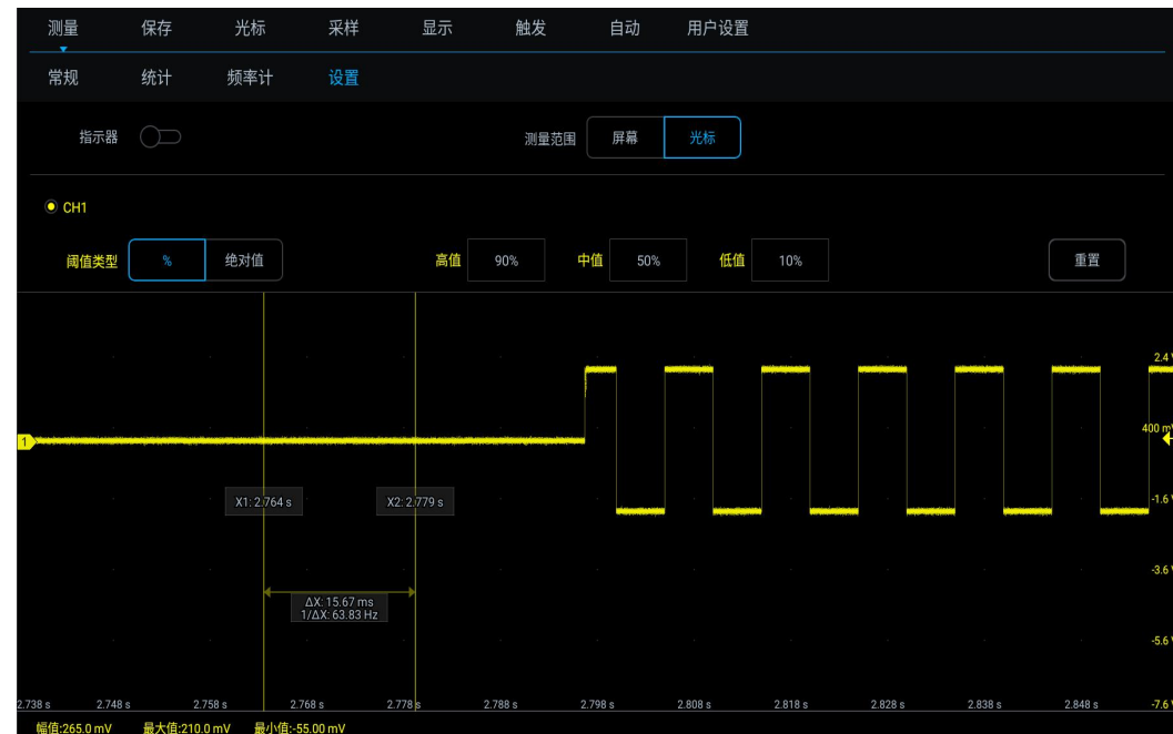
图 7-9 自动测量范围选为光标
