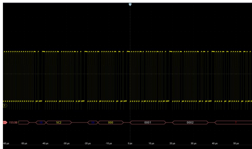
图 12-32 1553B 总线解码结果
