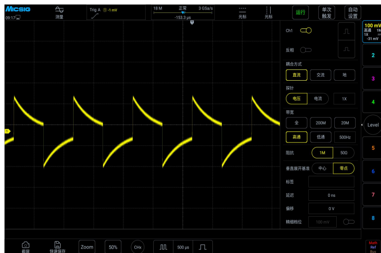
图5-12 20M带宽
