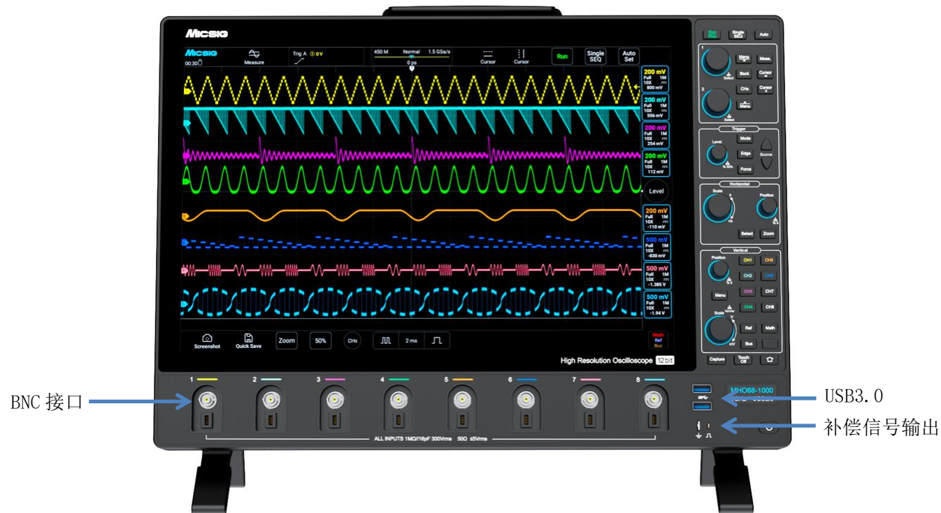
图 2-2 示波器正面
