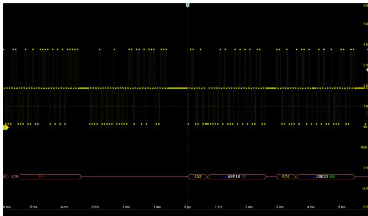
图 12-28 ARINC429 总线解码结果
