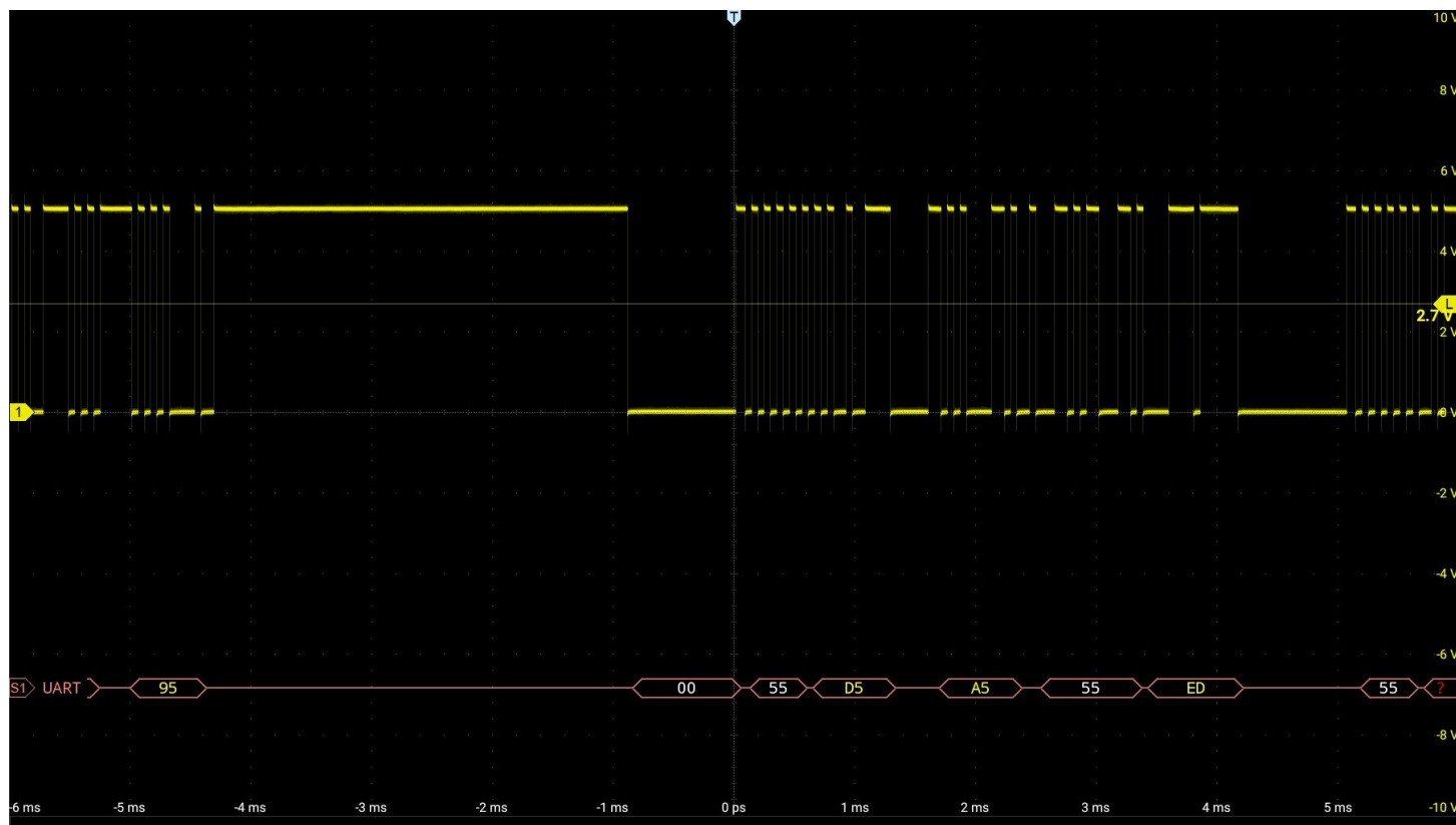
图 12-7 UART 解码阈值电平调节
