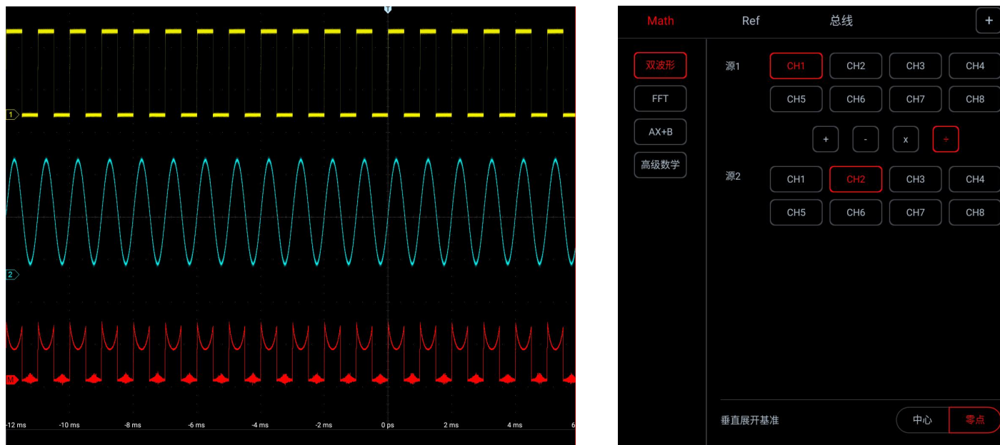
图 9-1 数学通道波形
