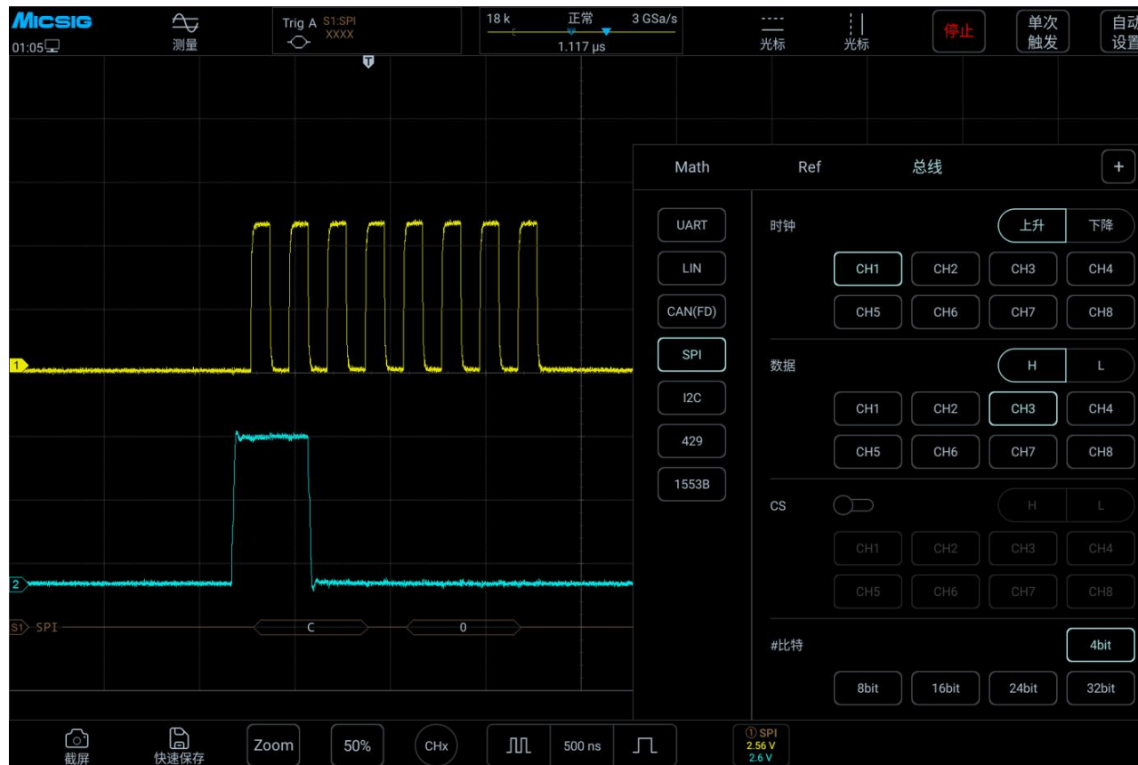
图 12-18 SPI 总线配置菜单
