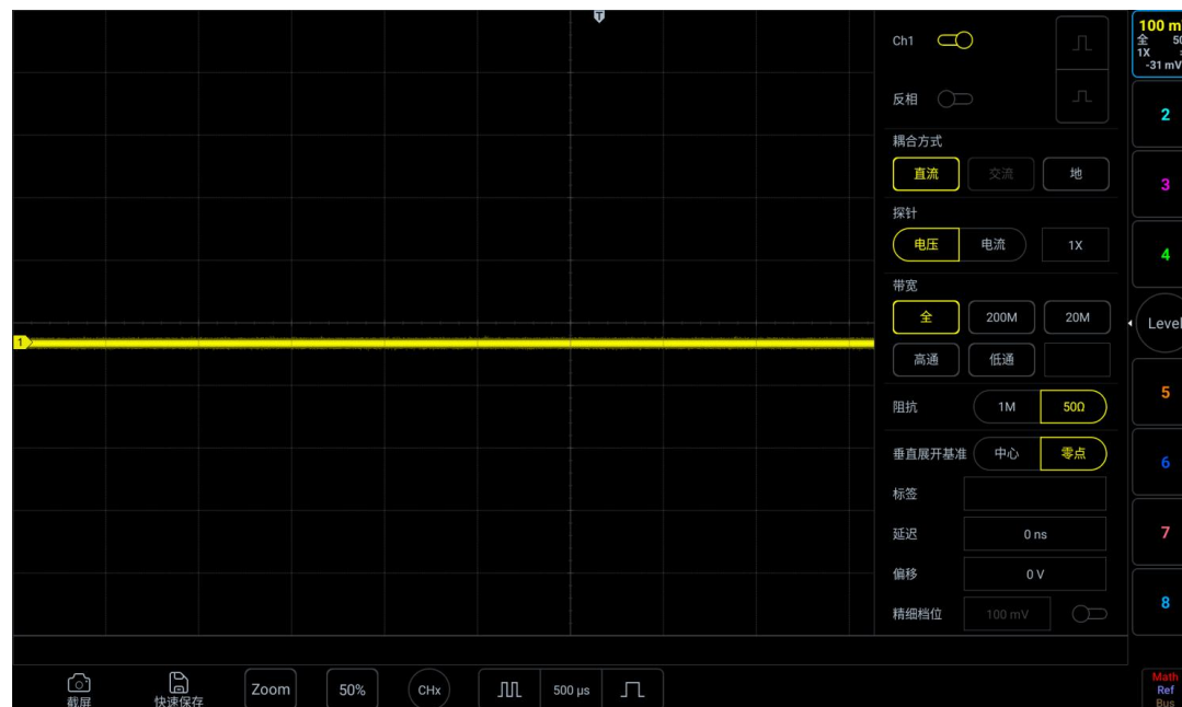
图5-18 通道输入阻抗
