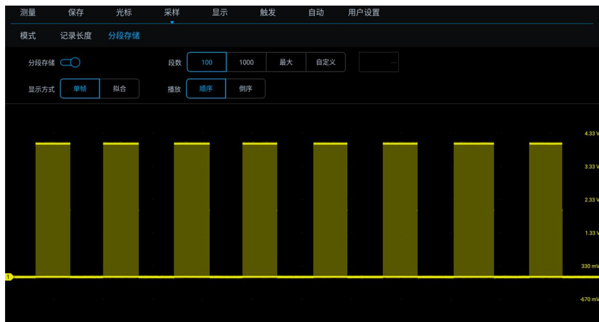
图 11-11 分段存储波形采集
