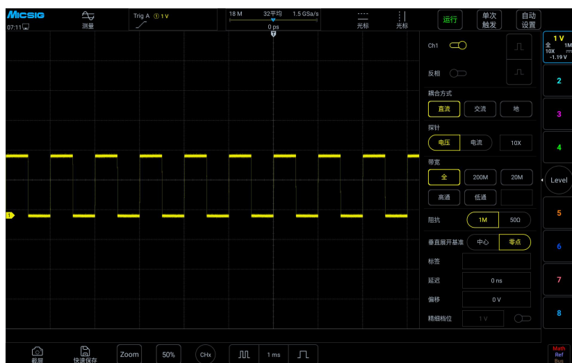
图5-7 DC耦合
