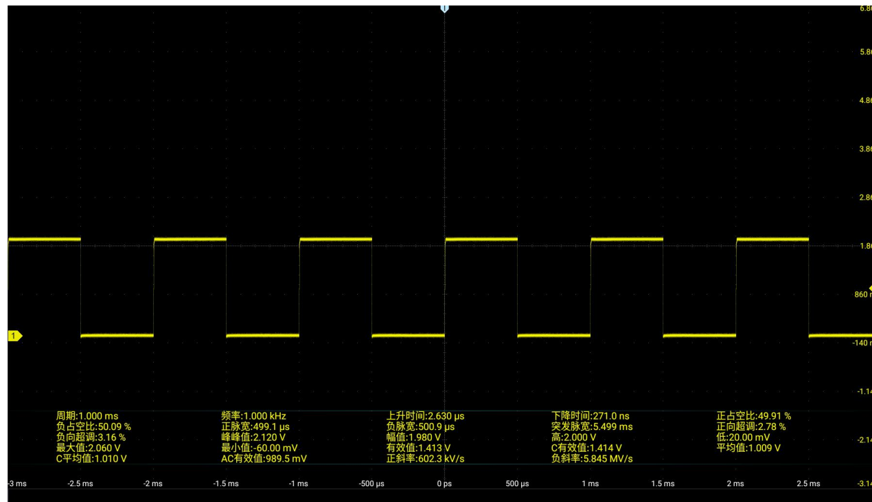
图 7-3 全部测量
