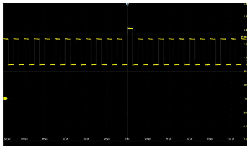
图 6-4 通过设置触发电平捕获到该异常信号
