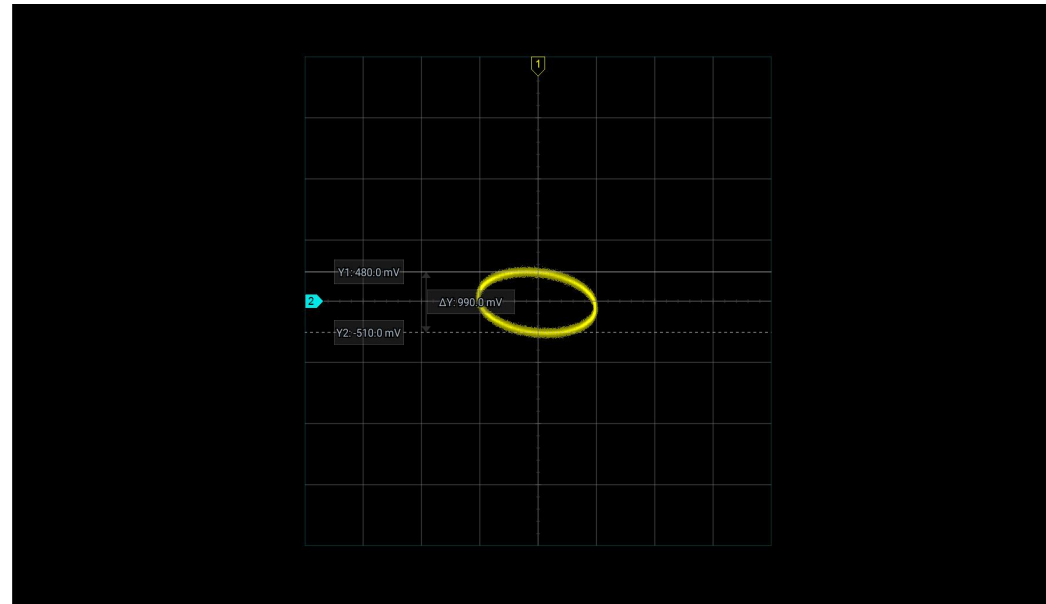
图 4-9 相差测量和使用光标
