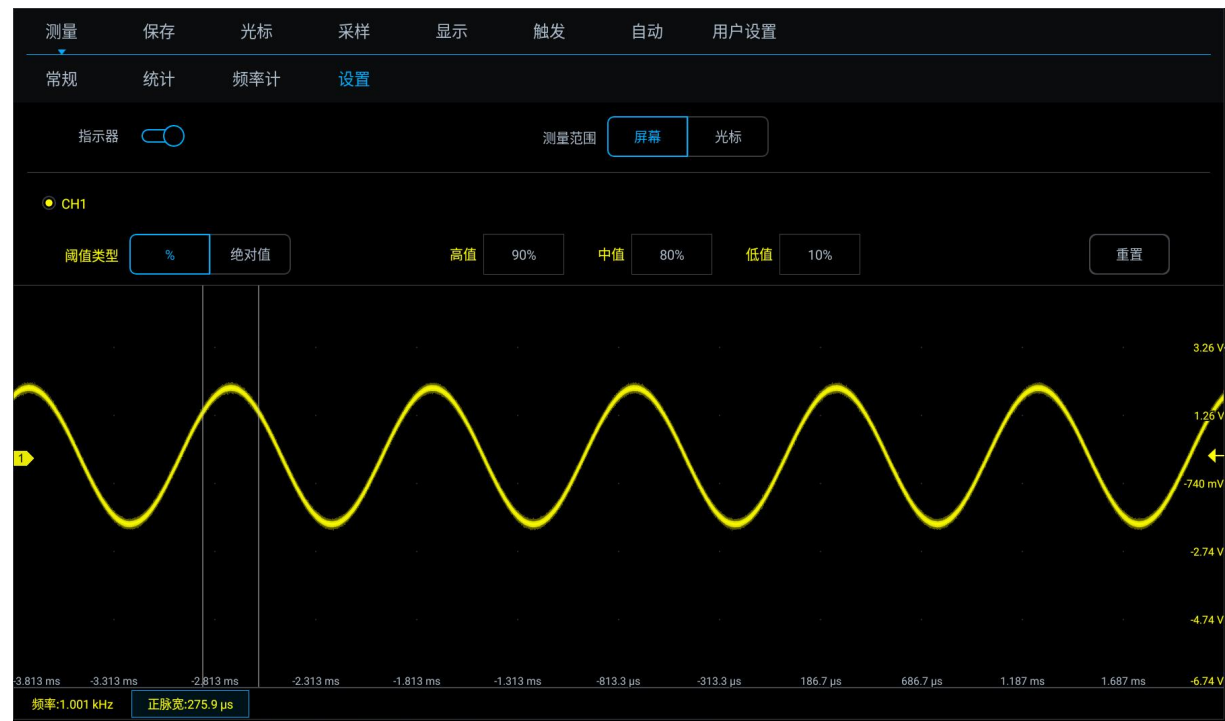
图 7-13 阈值中值设为 80%时的脉宽
