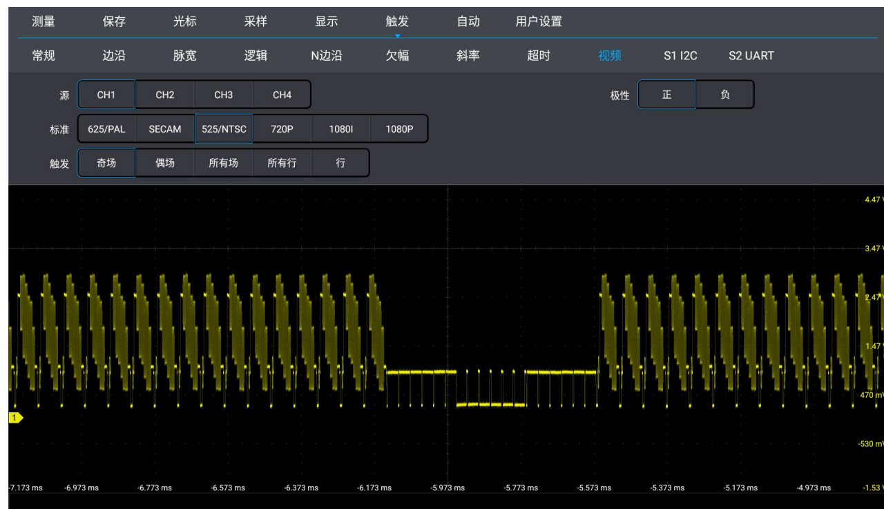
图 6-30 视频触发
