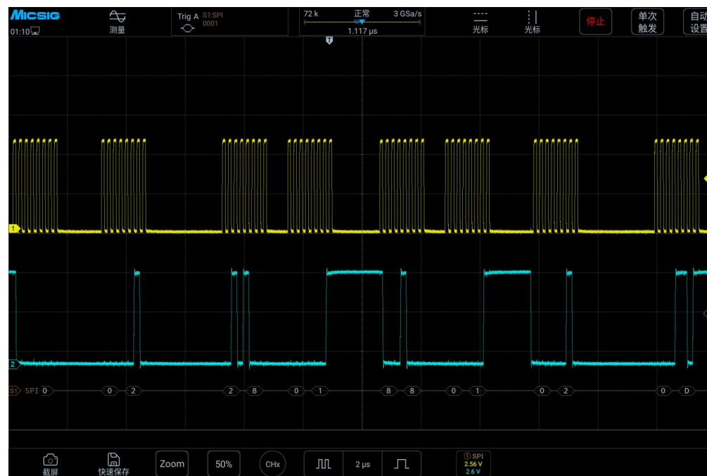
图 12-20 SPI 总线解码结果
