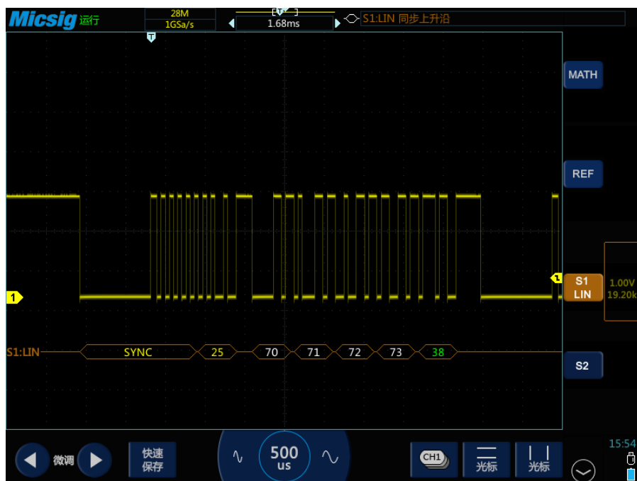
图13-11 LIN 图形界面
