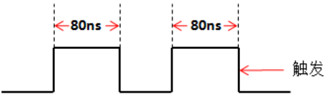
图5-15 触发时间 T=80\text{ns}
