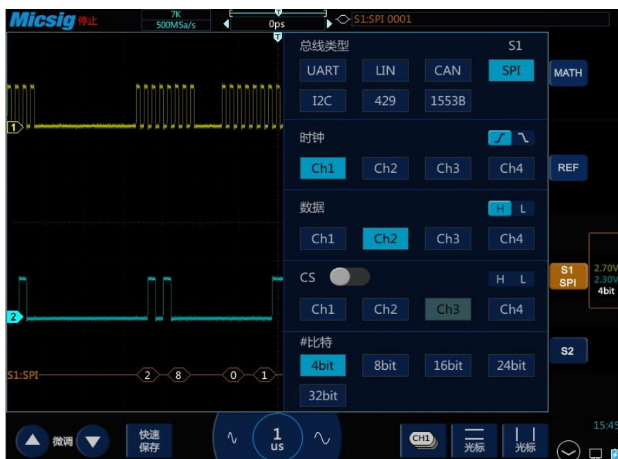
图13-17 SPI 总线配置菜单
