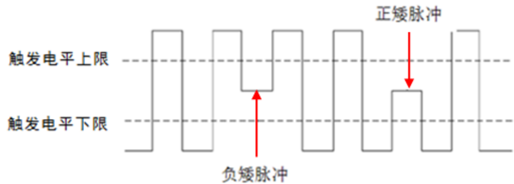
图5-21 欠幅触发
