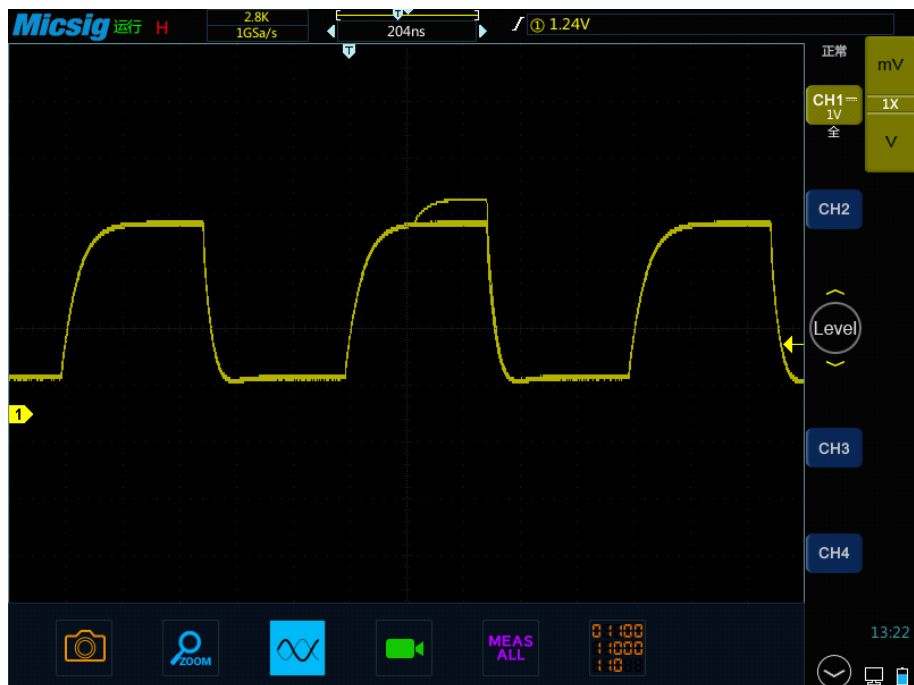
图9-5 高刷新模式
