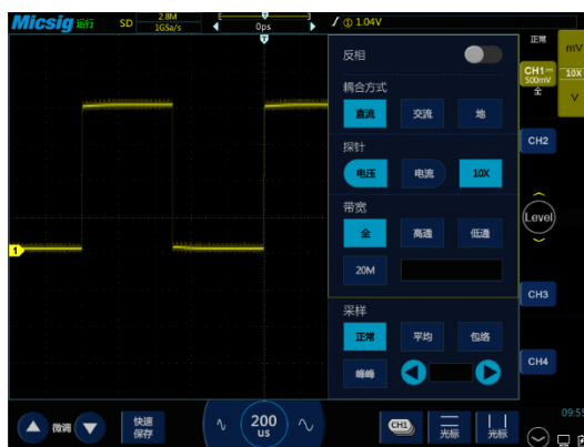
图4-9 全带宽
