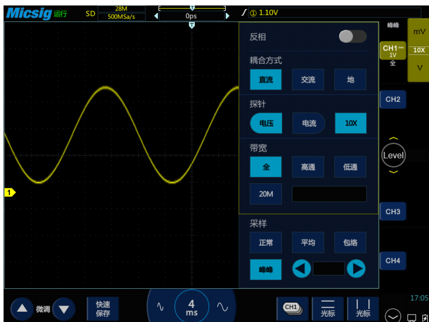
10-6 带毛刺的正弦波，峰值采样模式
