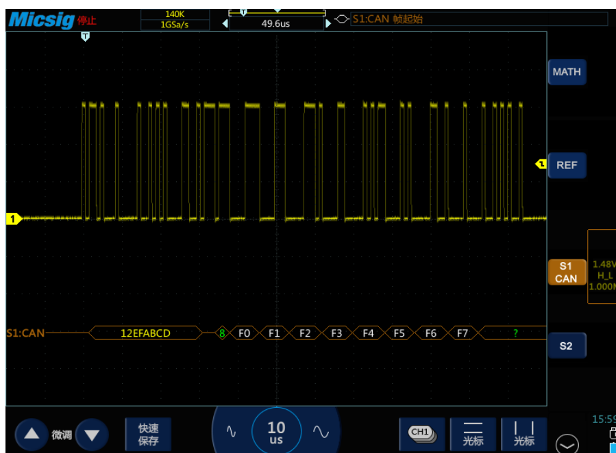
图13-15 CAN 图形界面
