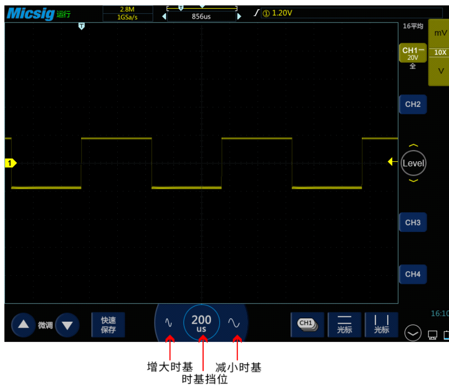
图3-3 调整水平时基
