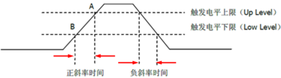
图5-23 正斜率时间/负斜率时间
