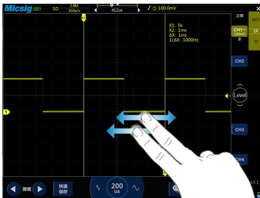
图6-9 光标测量脉冲宽度
