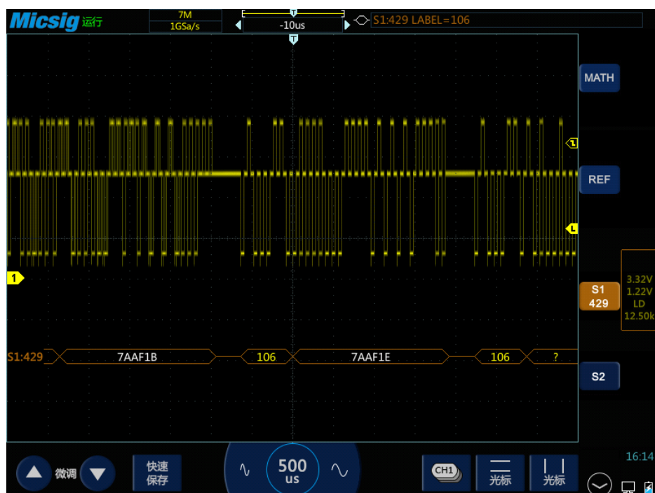
图13-27 ARINC429 图形界面
