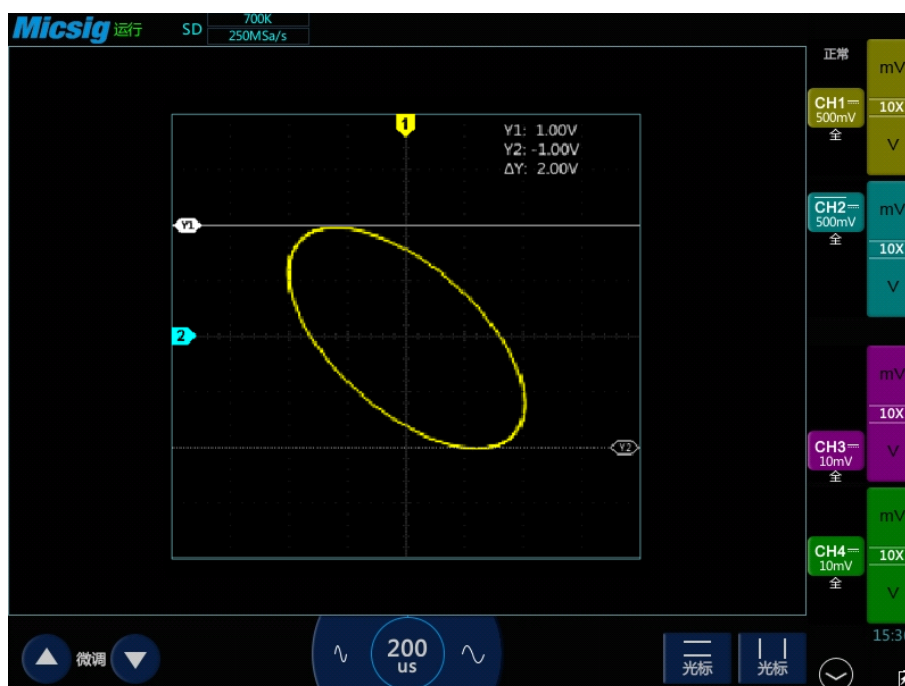
图6-10 XY 模式中，光标测量
