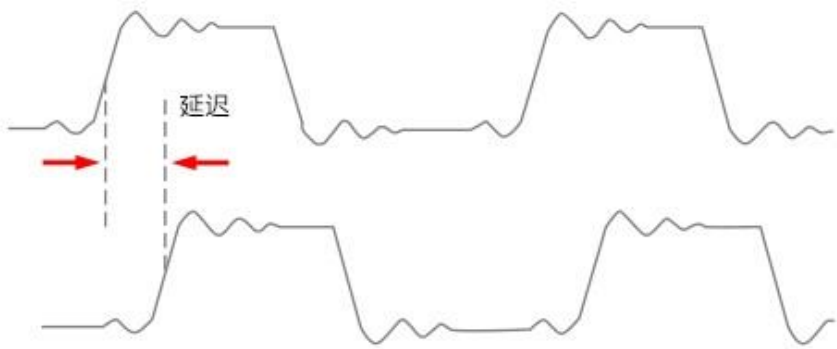
图6-4 延迟测量示意图
