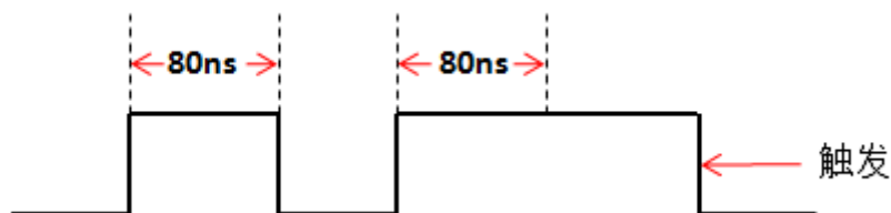
图5-14 触发时间 T > 80\text{ns}
