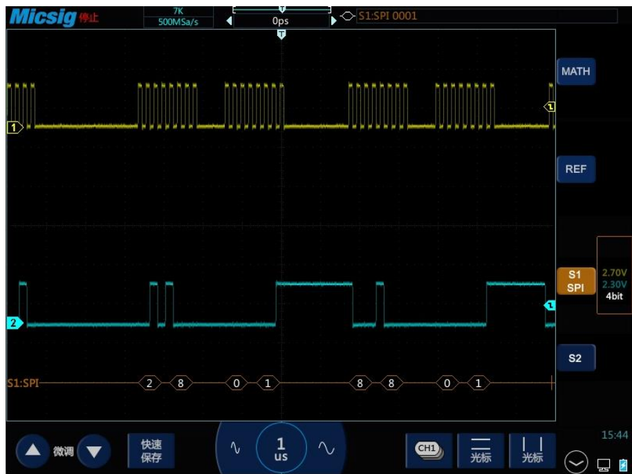
图13-19 SPI 图形界面
