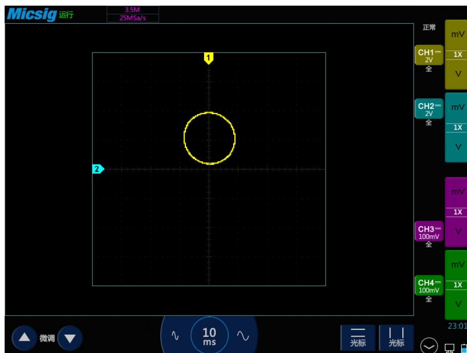
图3-7 XY 模式
