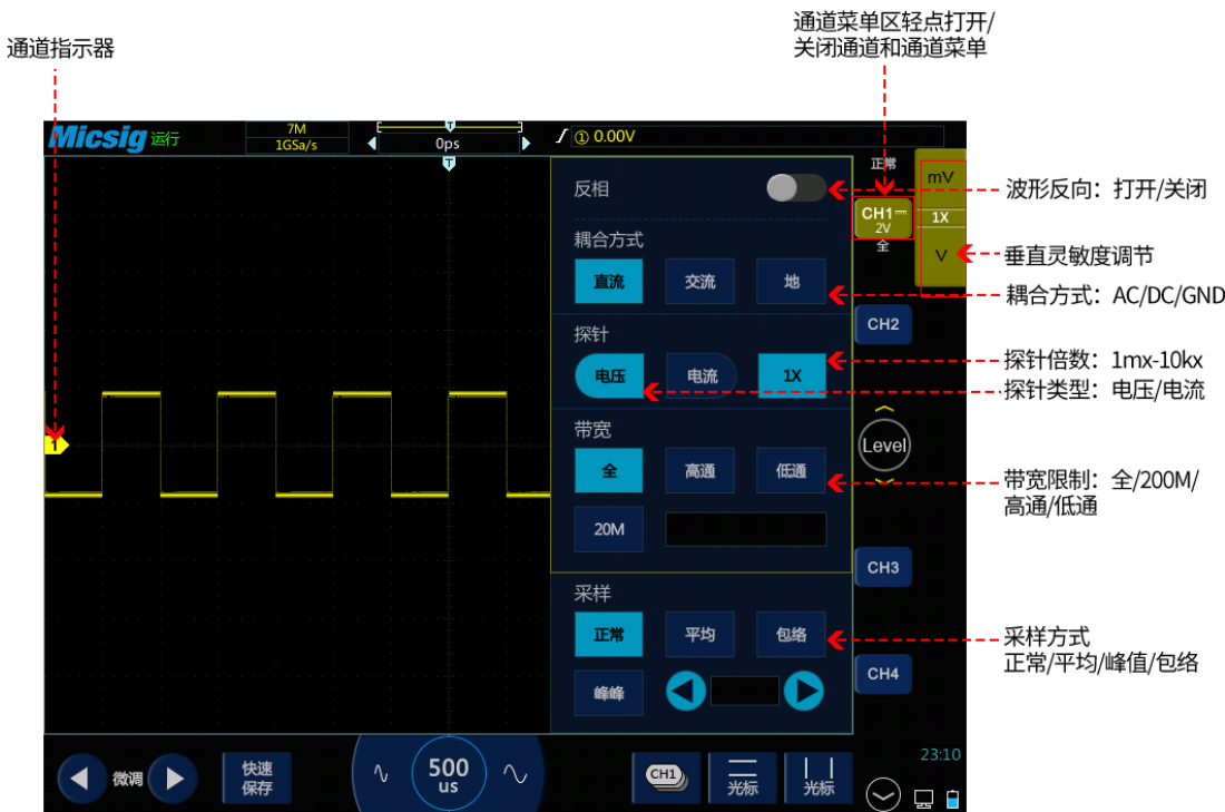
图4-1 通道菜单显示界面
