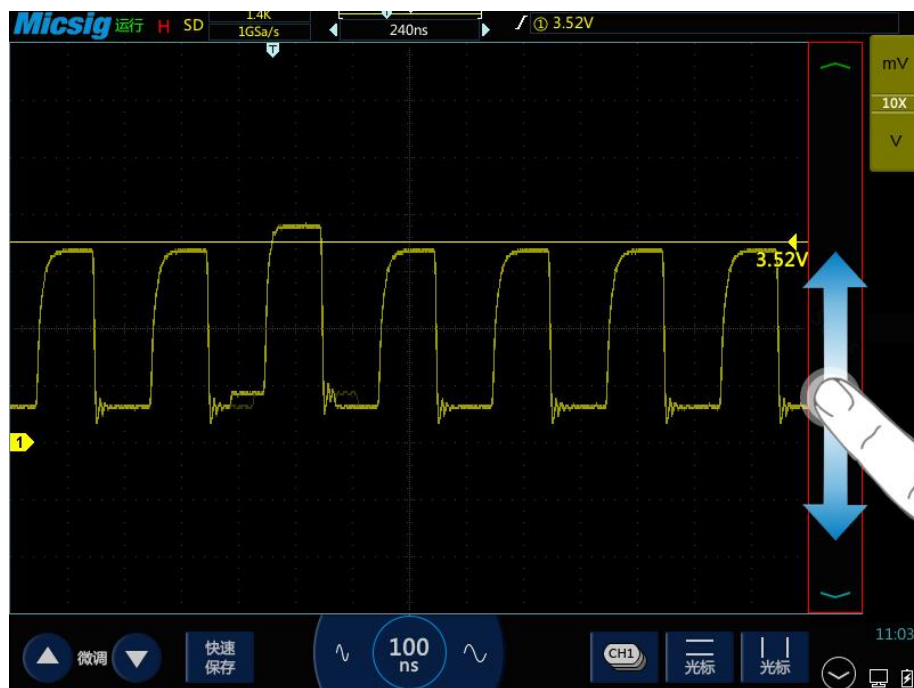
图5-3 通过设置触发电平捕获到该异常信号
