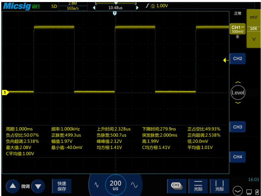
图6-3 全部测量
