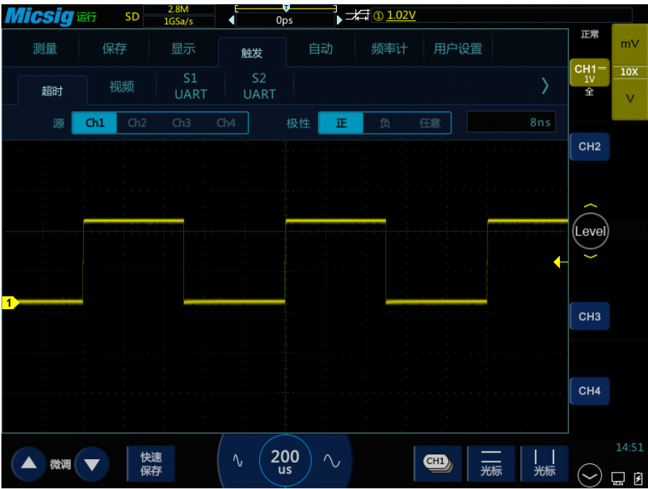
图5-26 超时触发
