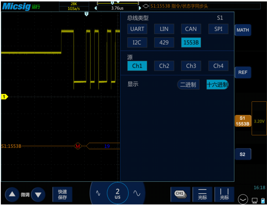
图13-29 1553B 总线配置菜单
