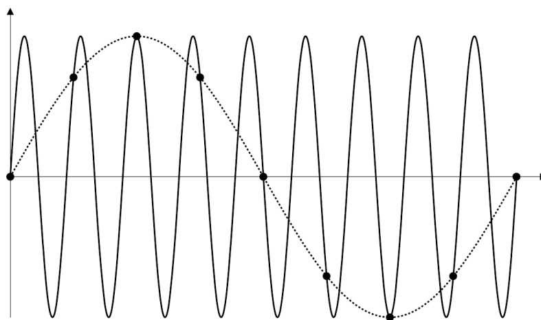
10-1 混叠
