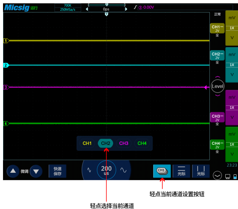
图4-4 使用当前通道选择按钮
