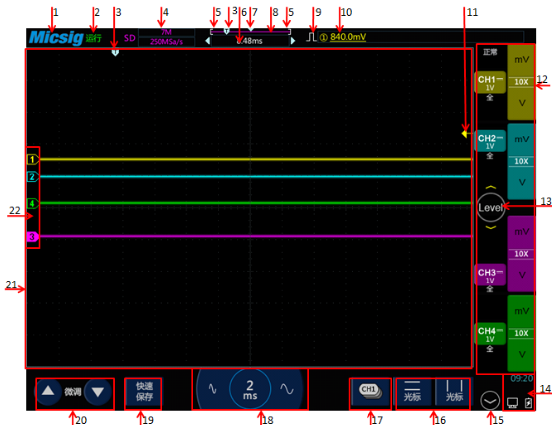
图2-4 示波器界面显示
