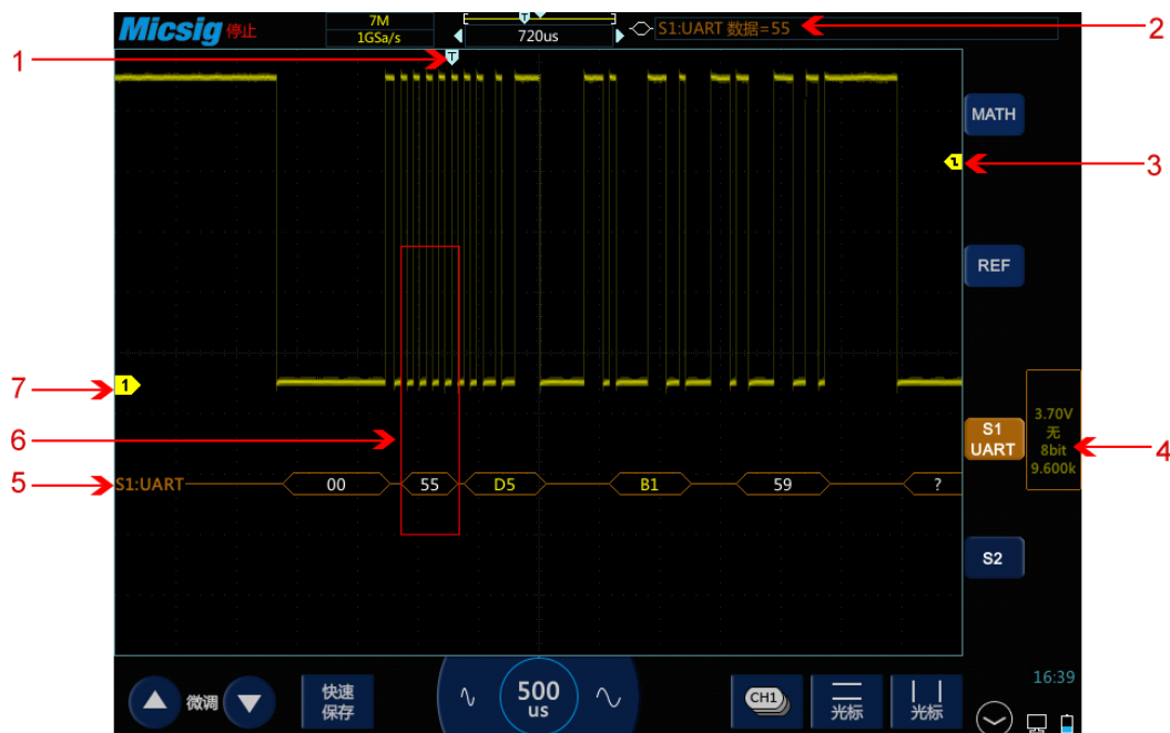
图13-7 UART 图形界面
