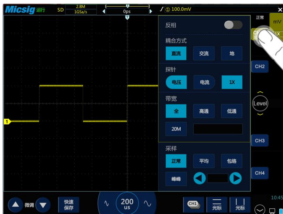
图4-6 通道切换图标及其菜单
