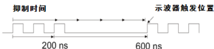
图5-7 触发抑制时间示意图说明
