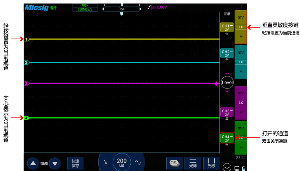
图4-3 通道的打开、关闭与切换
