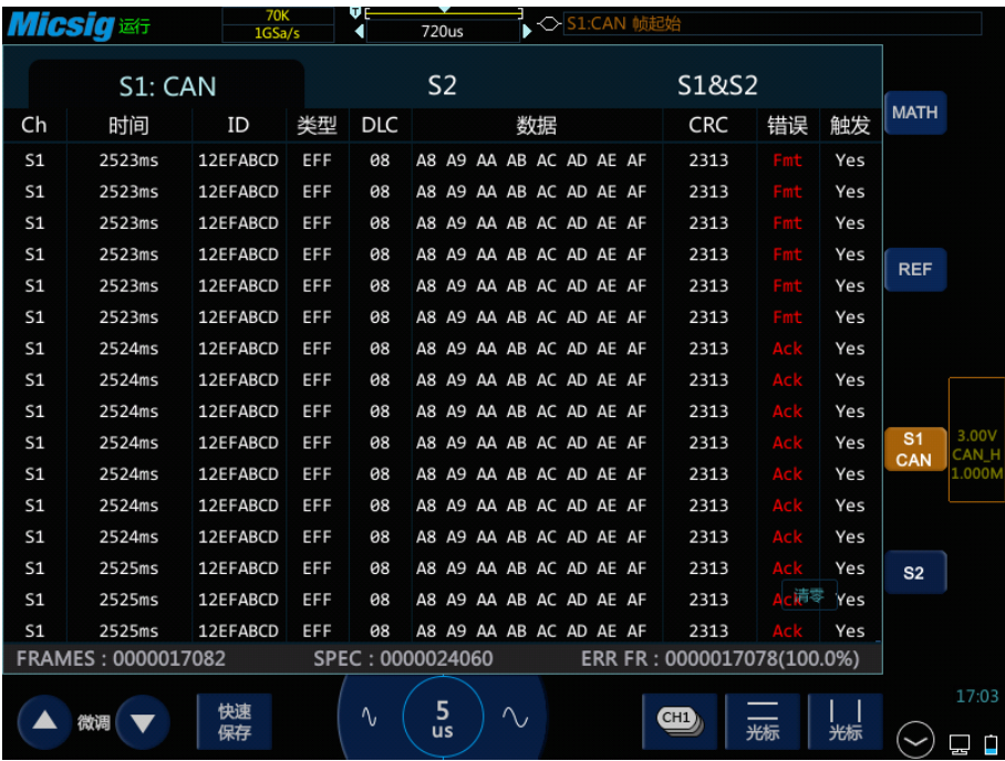
图13-16 CAN 文本界面
