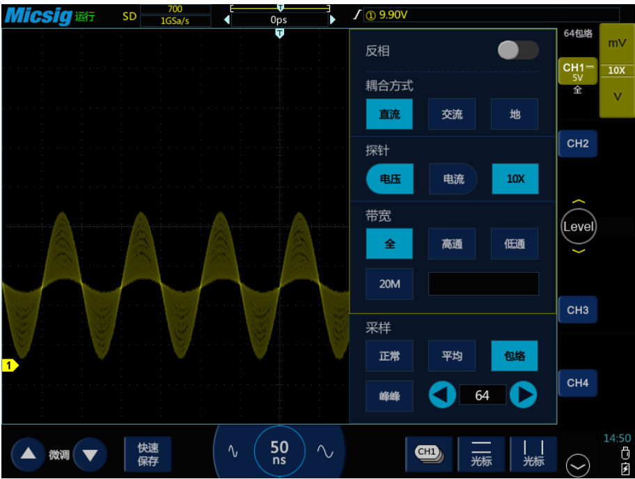
10-8 包络采样模式（64）下的调幅信号
