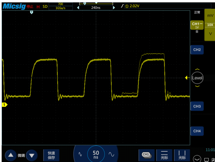
图5-2 周期信号中有异常信号
