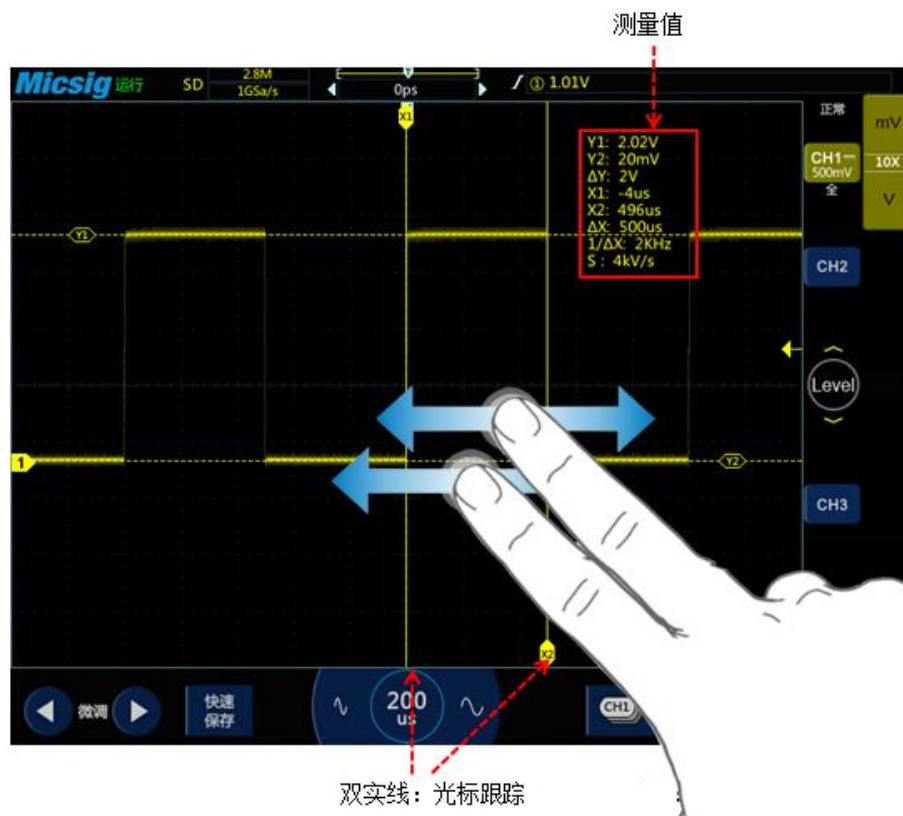
图6-7 光标测量说明
