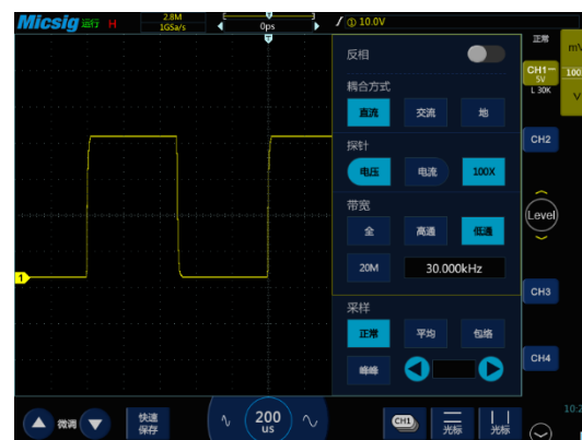
图4-12 低通
