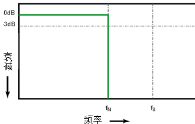
10-2 理论上的砖墙频率响应
