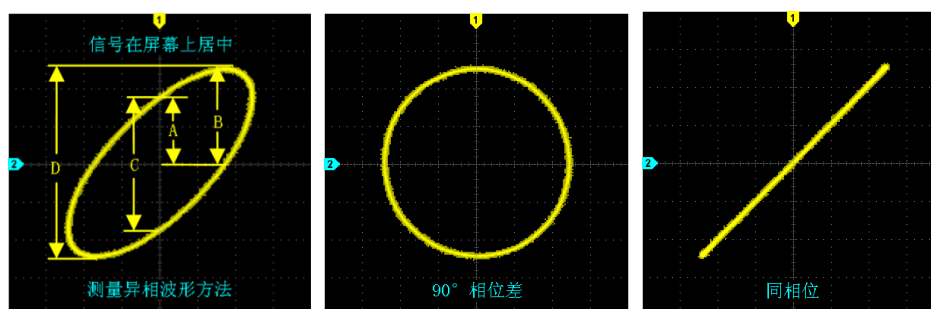
图3-8 XY 时基模式信号，在显示屏上居中
