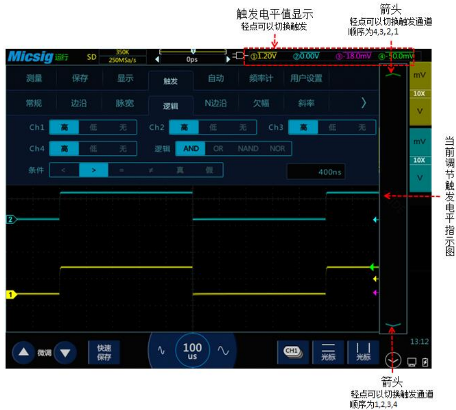
图5-19 触发电平调节
