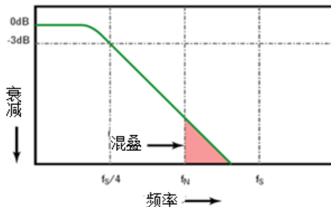
10-3 采样率和示波器带宽
