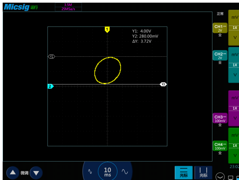
图3-9 相差测量和使用光标
