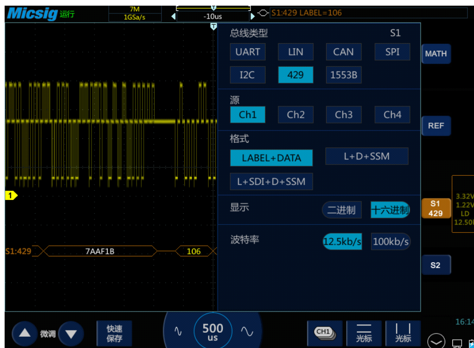
图13-25 ARINC429 总线配置菜单
