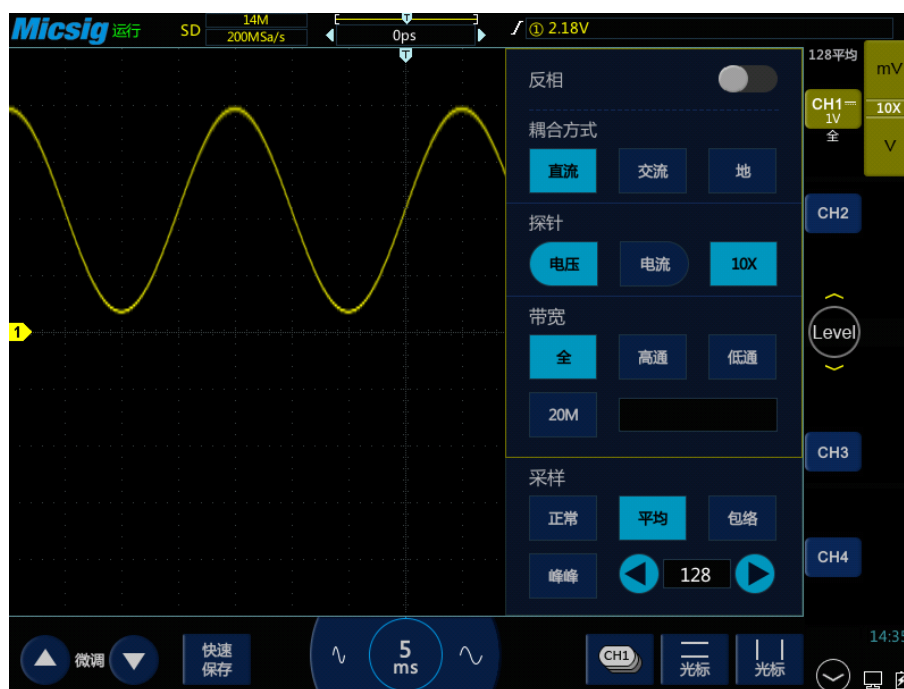
10-7 选择平均采样模式后的波形，平均数 128
