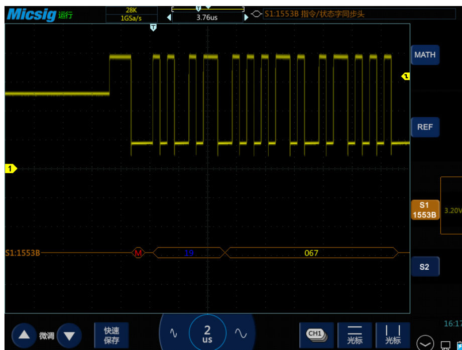
图13-31 1553B 图形界面
