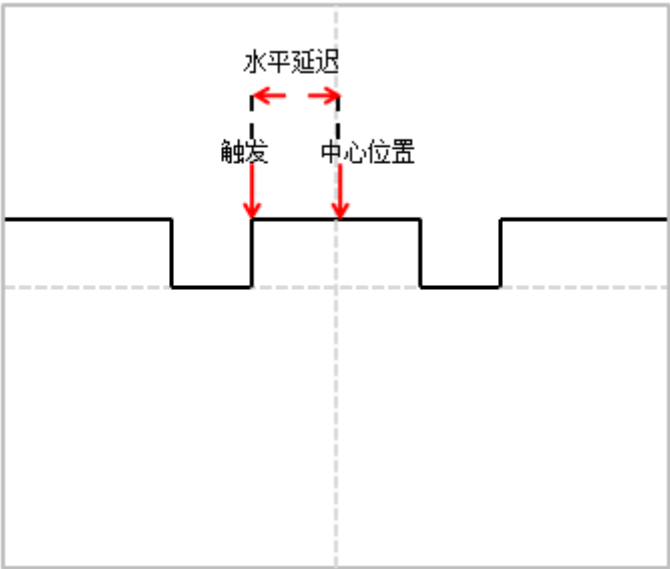
图5-5 水平延迟
