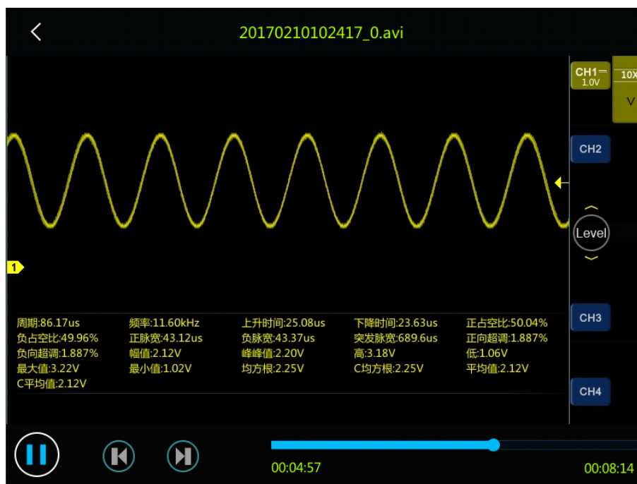
图11-12 视频回放界面
