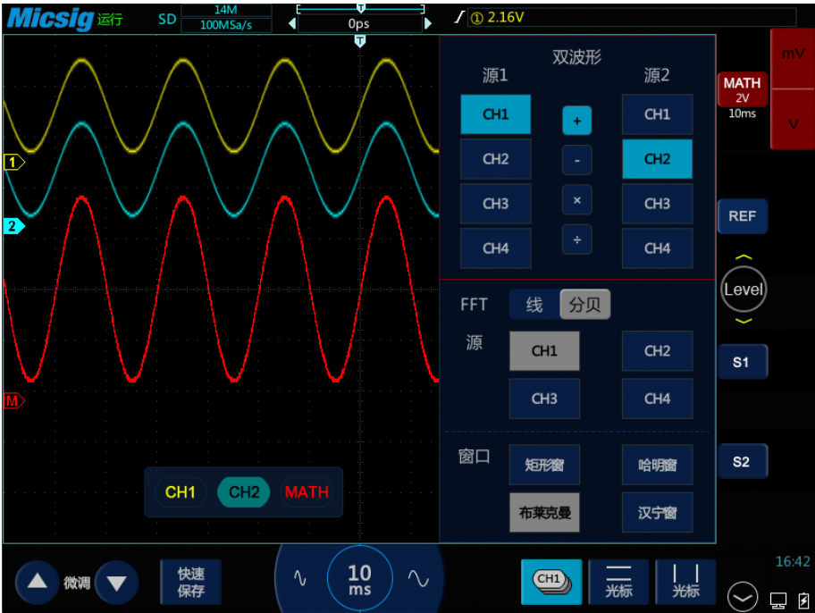
图8-2 通道 1 加通道 2 数学运算示图
