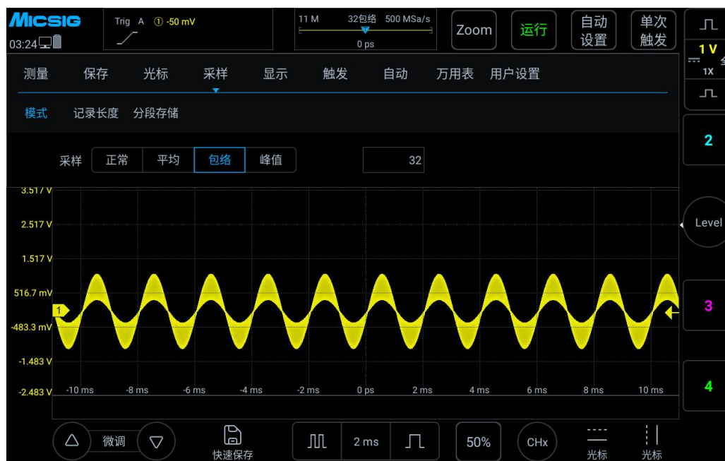
图 13-8 包络采样模式（32）下的调幅信号
