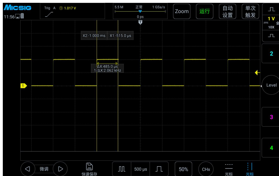
图 8-17 光标测量脉冲宽度
