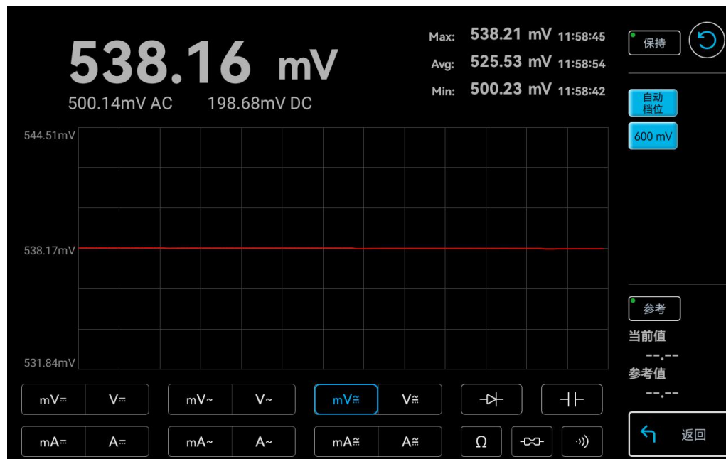
图 9-8 交直流电压测量 mV
