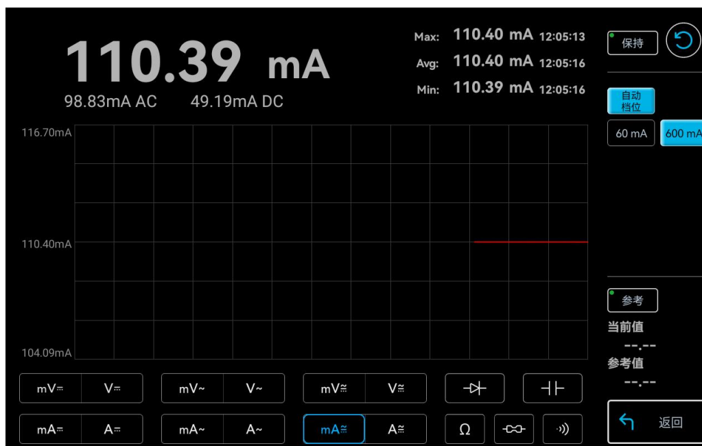
图 9-14 交直流电流测量 mA
