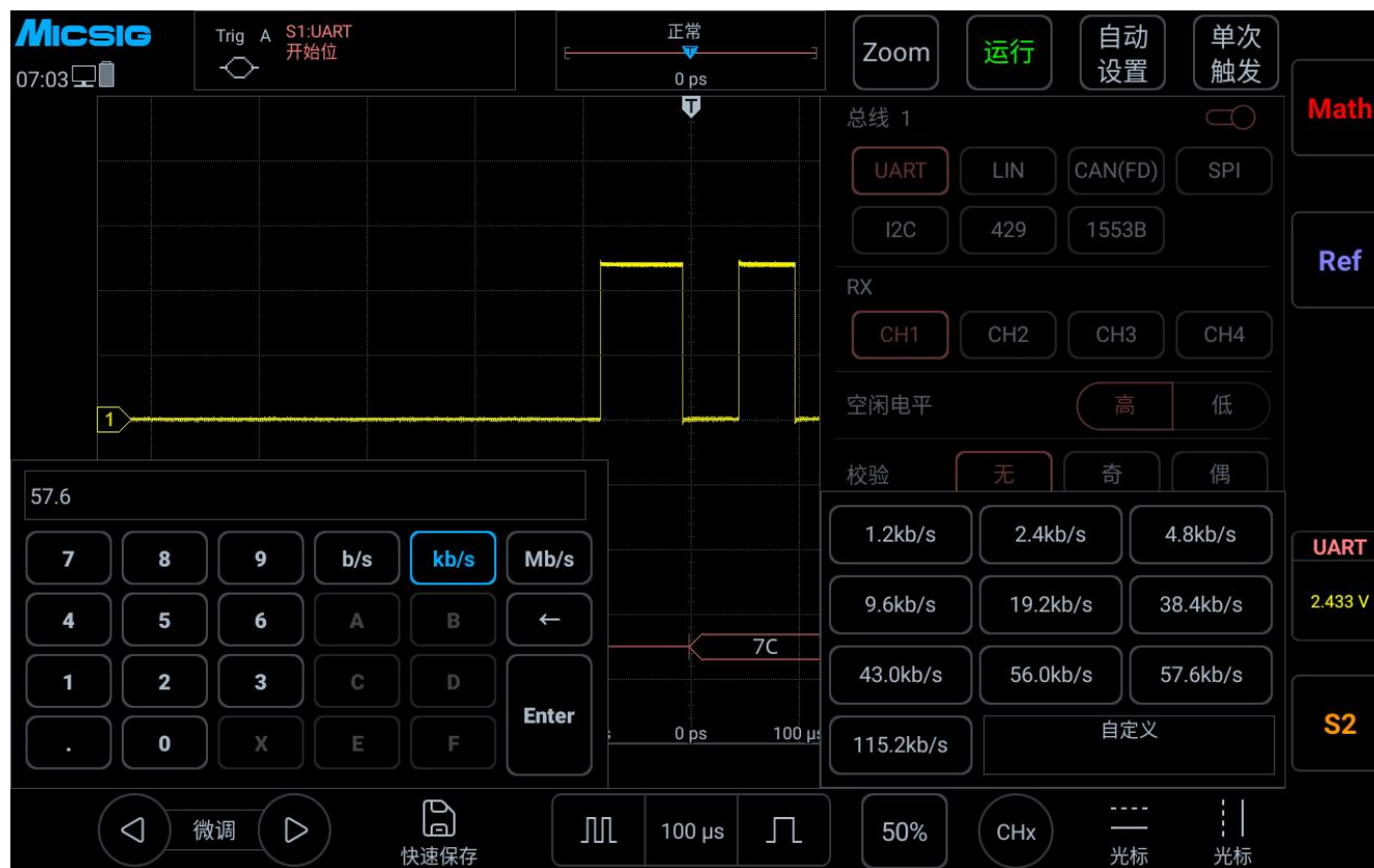
图 14-5 波特率自定义设置
