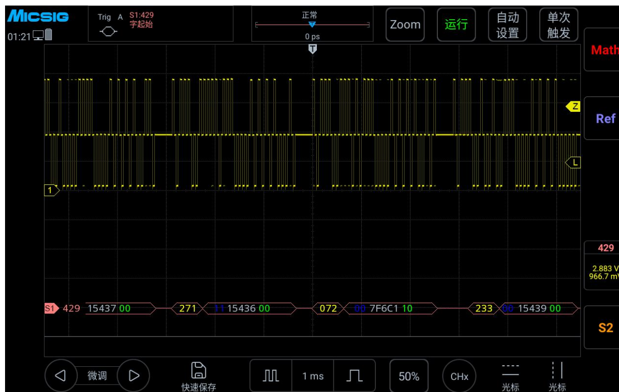
图 14-28 ARINC429 图形界面
