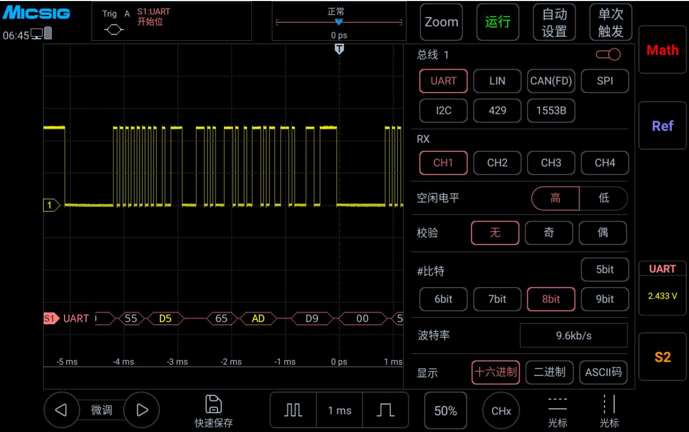
图 14-1 总线类型选择菜单
