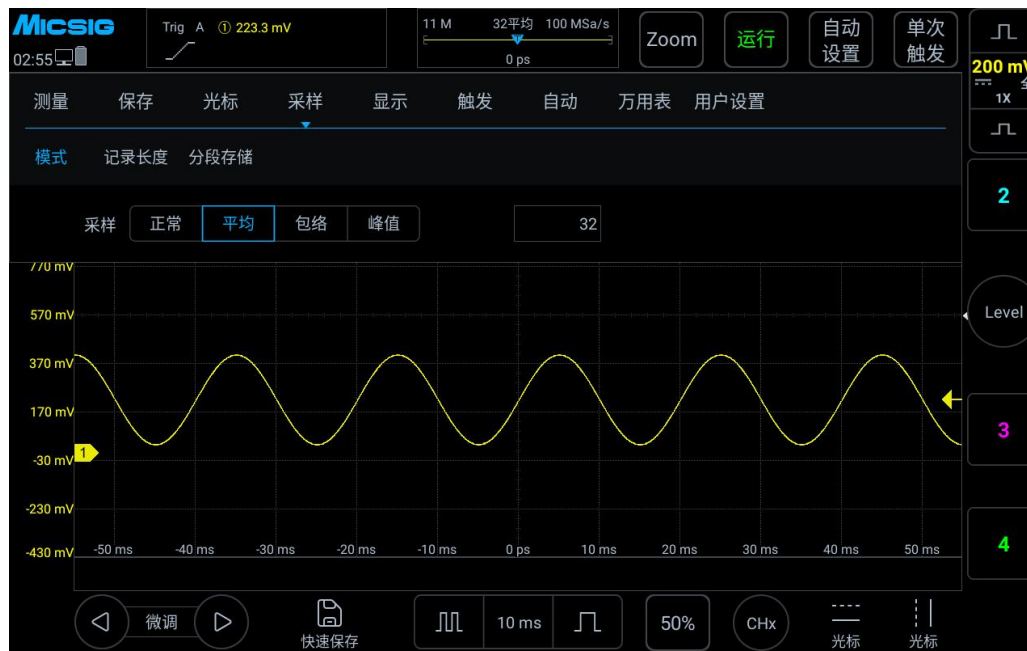
图 13-5 选择平均采样模式后的波形，平均数 32
