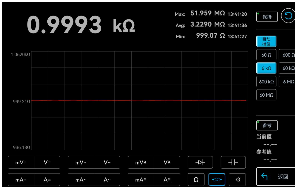
图 9-16 在线电阻测量
