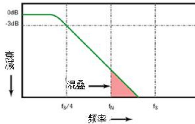
图 13-3 采样率和示波器带宽
