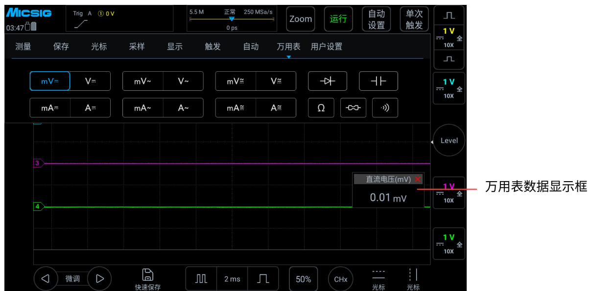
图 9-1 万用表数据显示框
