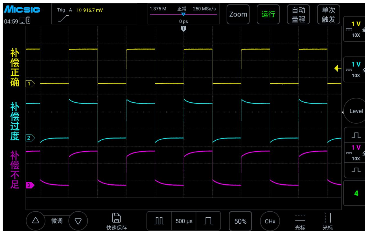
图 2-12 探头补偿
