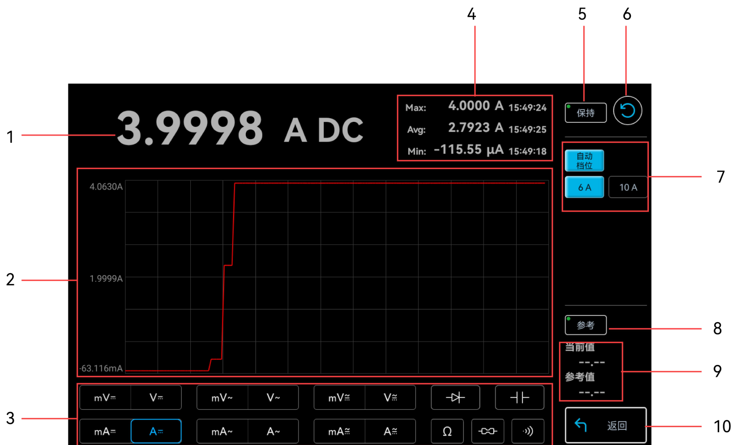
图 9-2 万用表界面
