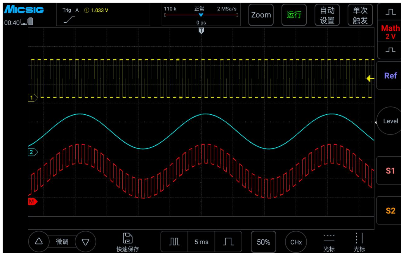
图 11-2 通道 1 加通道 2 数学运算示图
