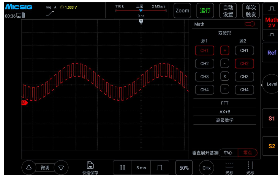
图 11-1 数学通道波形
