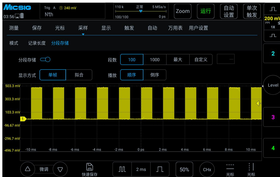
图 13-11 分段存储波形采集
