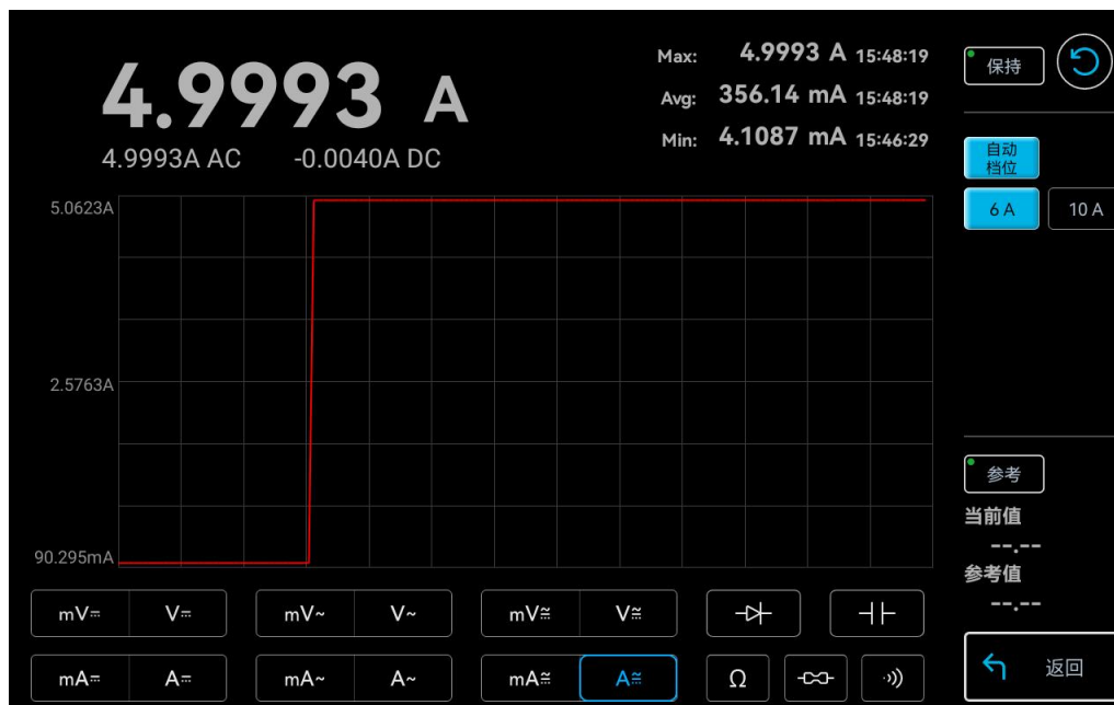
图 9-11 交直流电流测量 A
