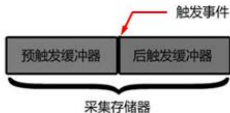
图 7-6 采集存储器的概念演示
