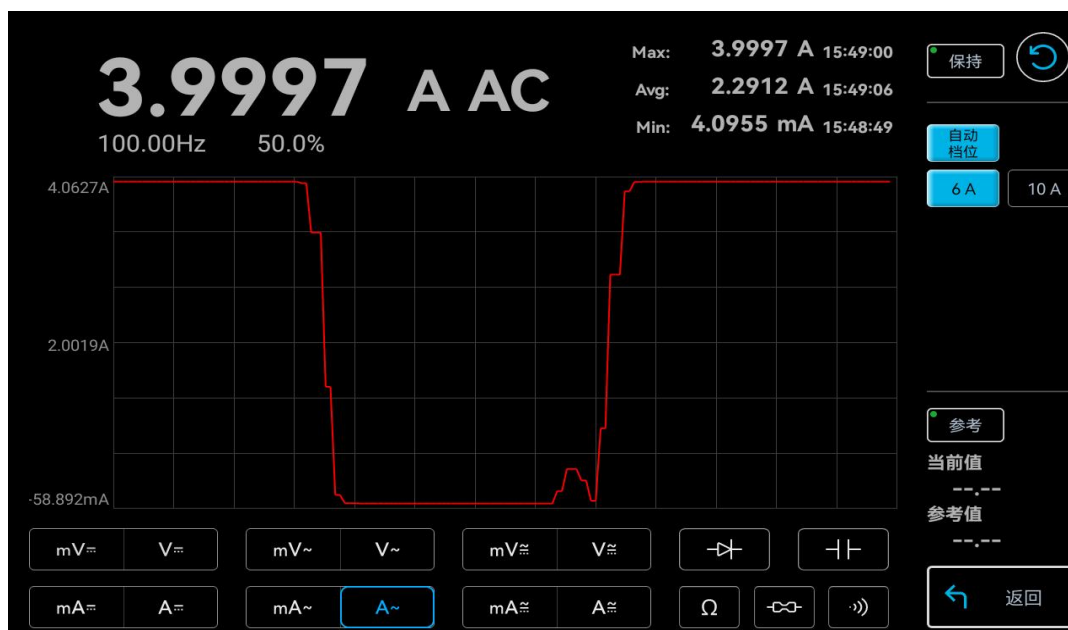
图 9-10 交流电流测量 A
