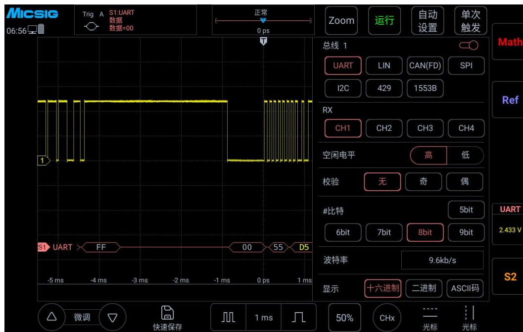
图 14-4 UART 总线配置菜单
