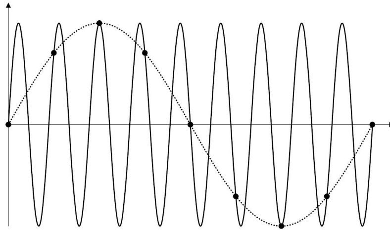
图 13-1 混叠
