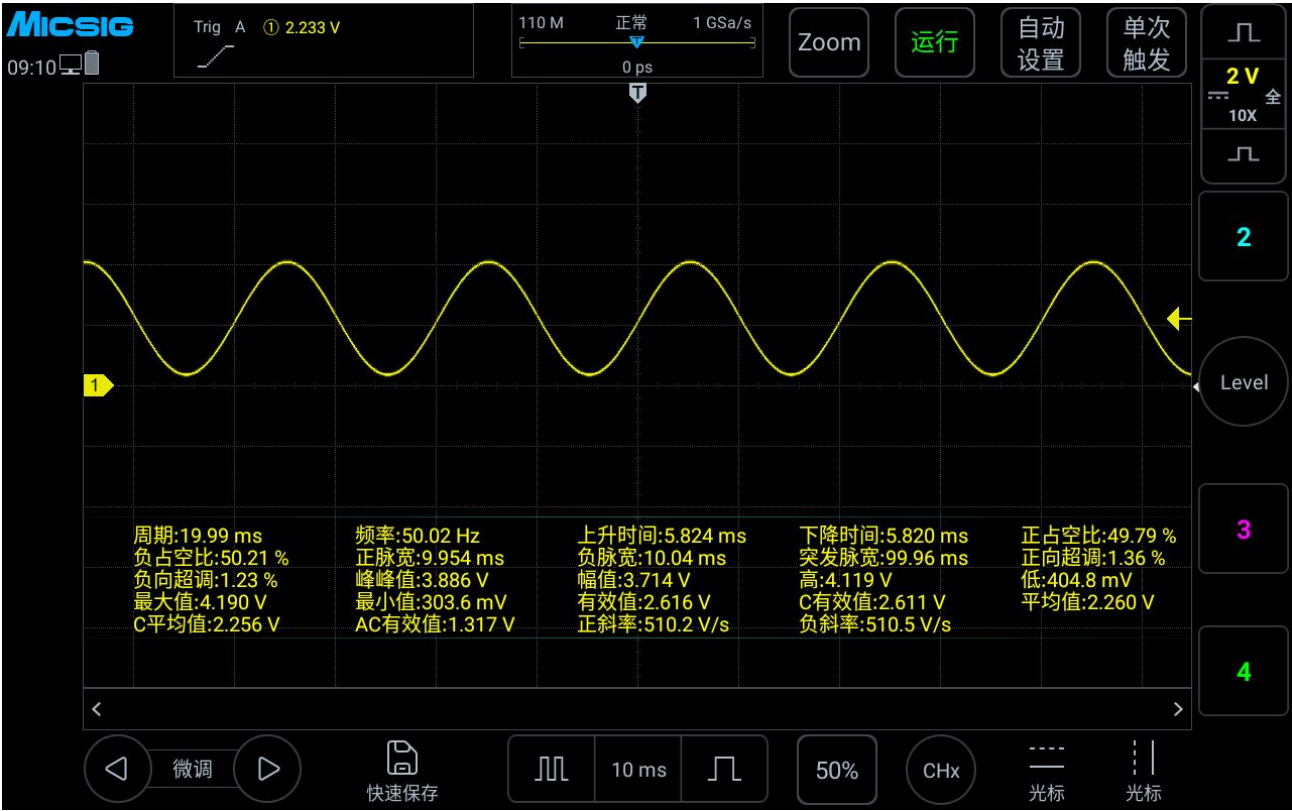
图 8-3 全部测量
