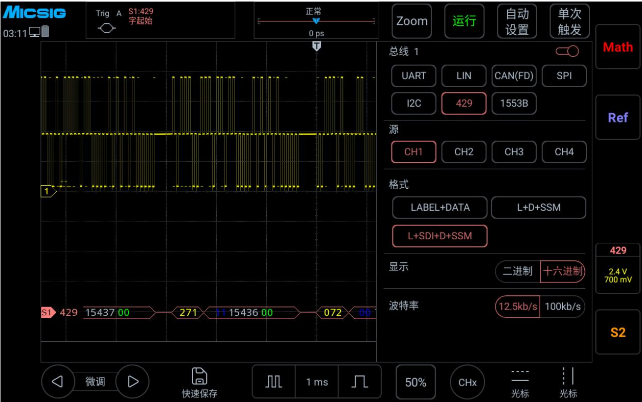
图 14-26 ARINC429 总线配置菜单
