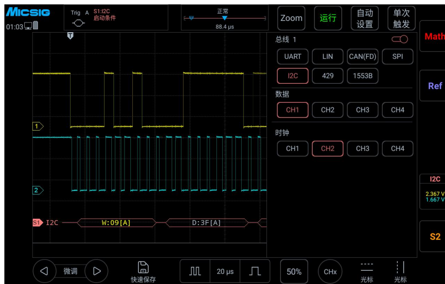
图 14-22 I2C 总线配置菜单
