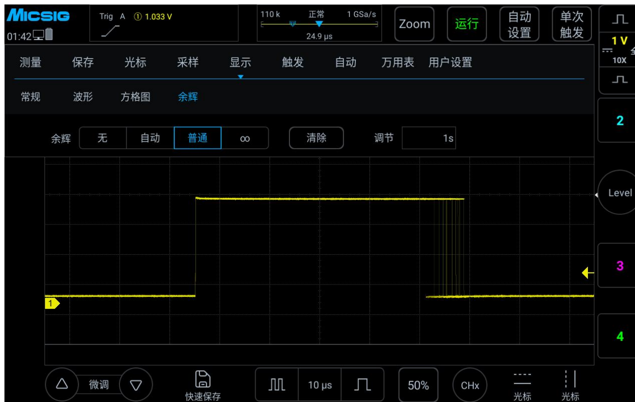
图 12-4 余辉时间调节
