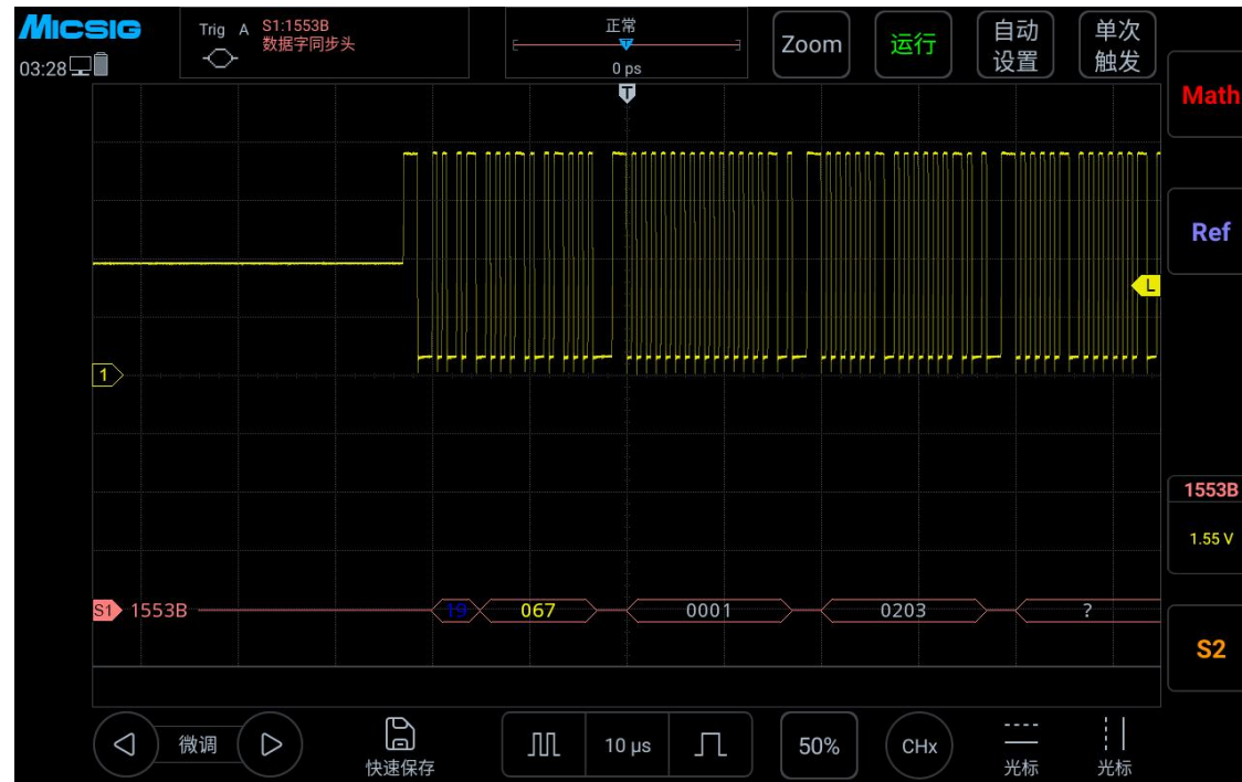
图 14-32 1553B 图形界面
