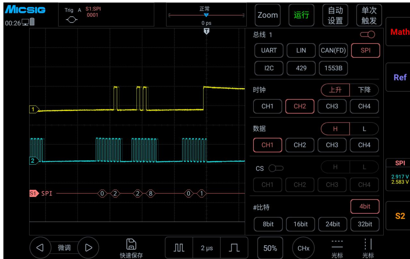
图 14-18 SPI 总线配置菜单
