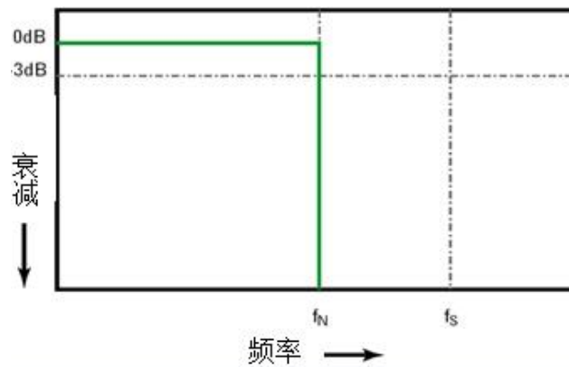
图 13-2 理论上的砖墙频率响应
