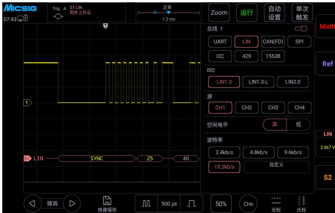
图 14-10 LIN 总线配置菜单
