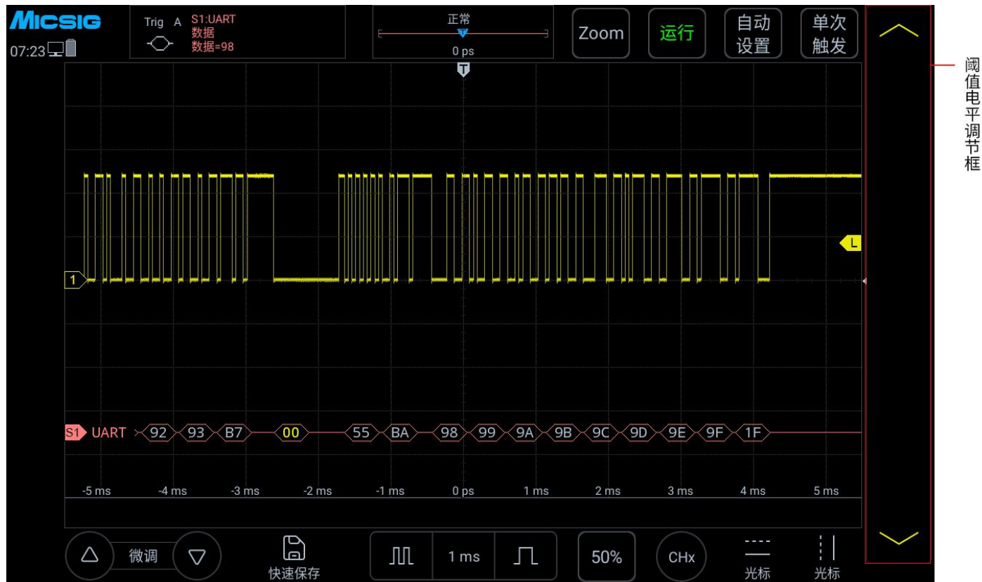
图 14-7 UART 解码电平调节
