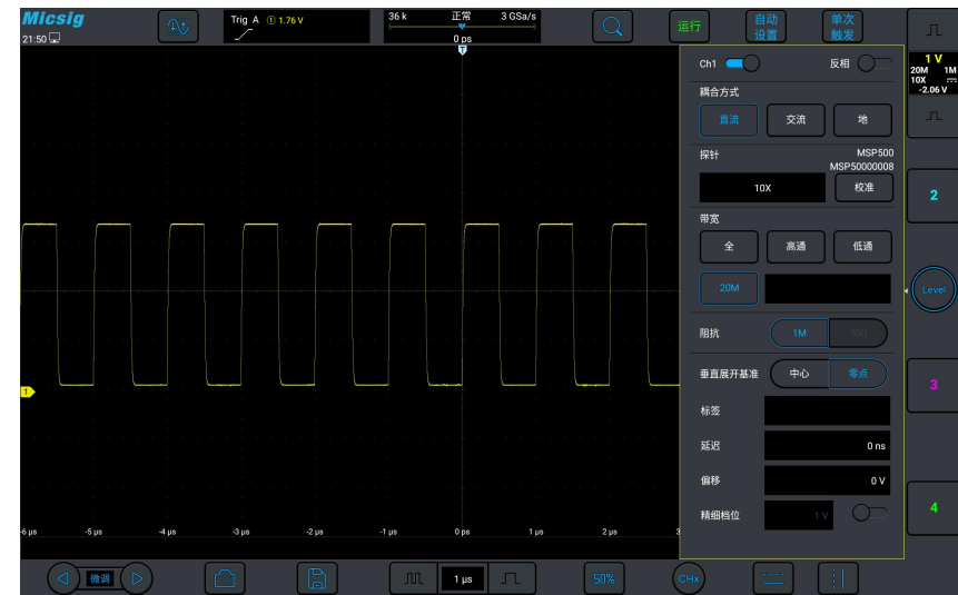
图5-11 20M带宽
