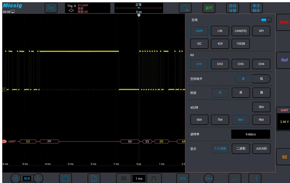
图 12-4 UART 总线配置菜单
