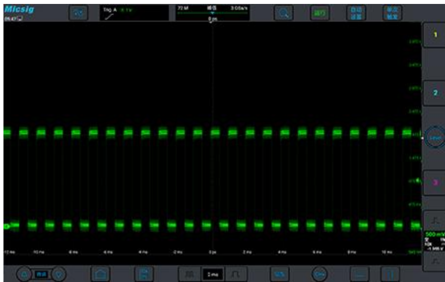
图 11-5 带毛刺的波形，峰值采样模式
