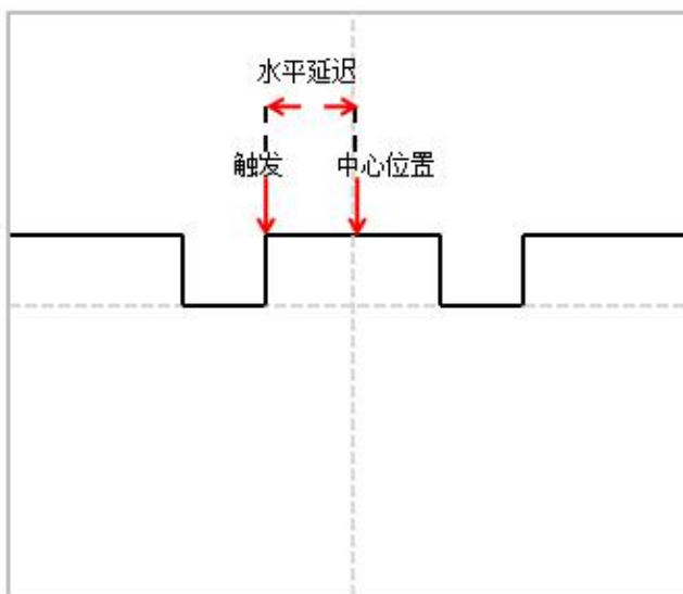
图 6-7 水平延迟
