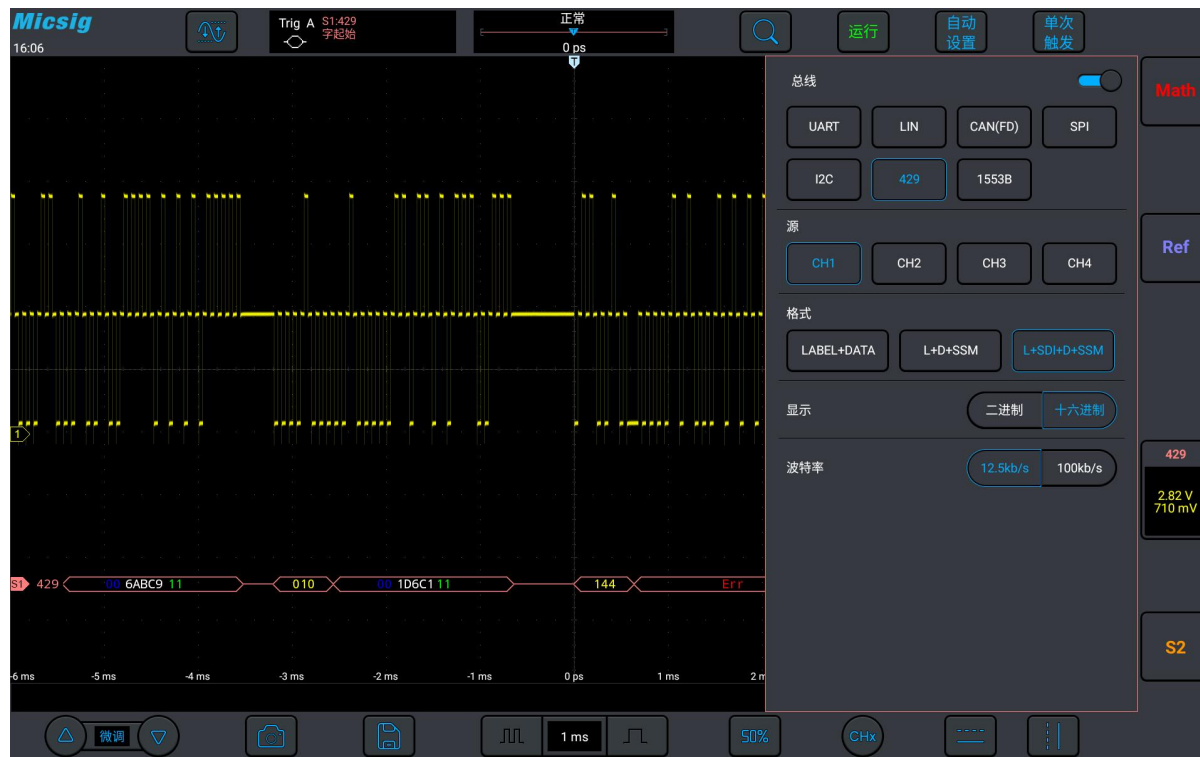
图 12-26 ARINC429 总线配置菜单
