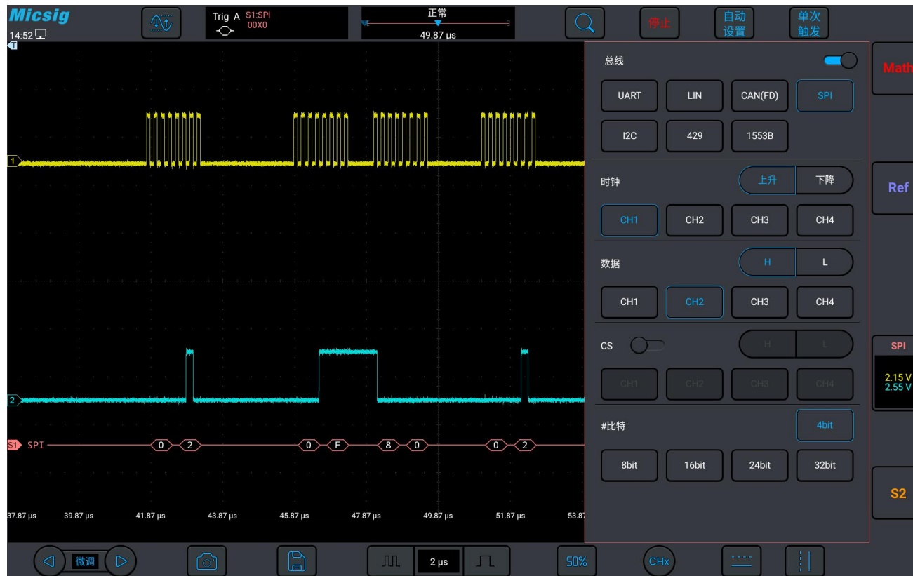
图 12-18 SPI 总线配置菜单
