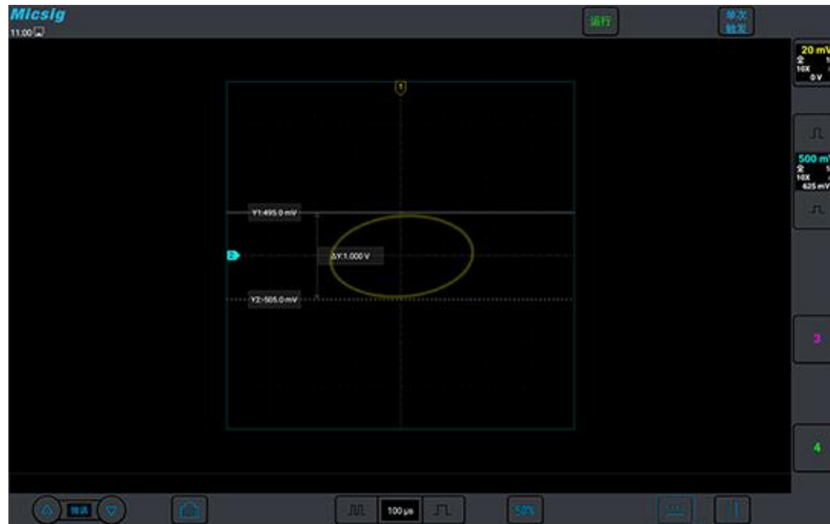
图 4-9 相差测量和使用光标
