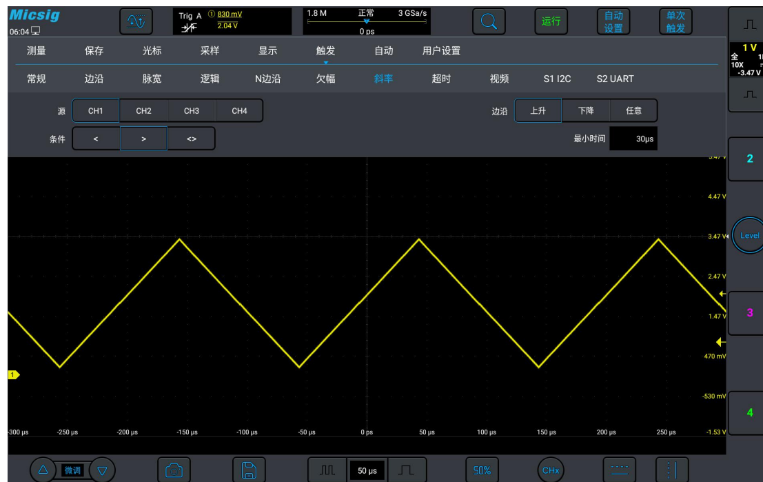
图 6-27 斜率触发设置菜单
