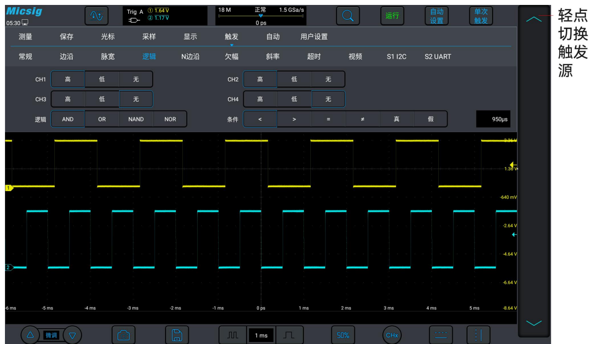
图 6-22 切换触发电平通道
