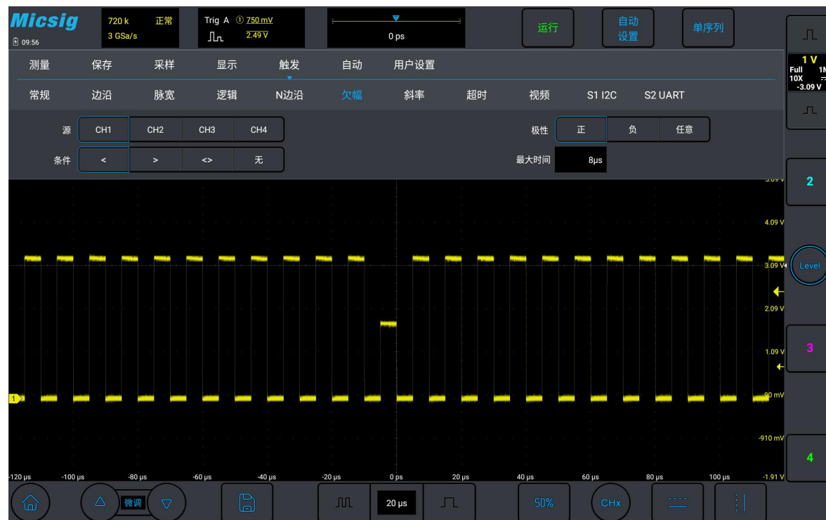
图 6-25 欠幅触发设置菜单
