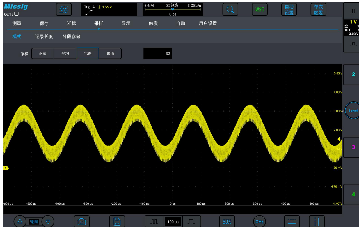
图 11-8 包络采样模式
