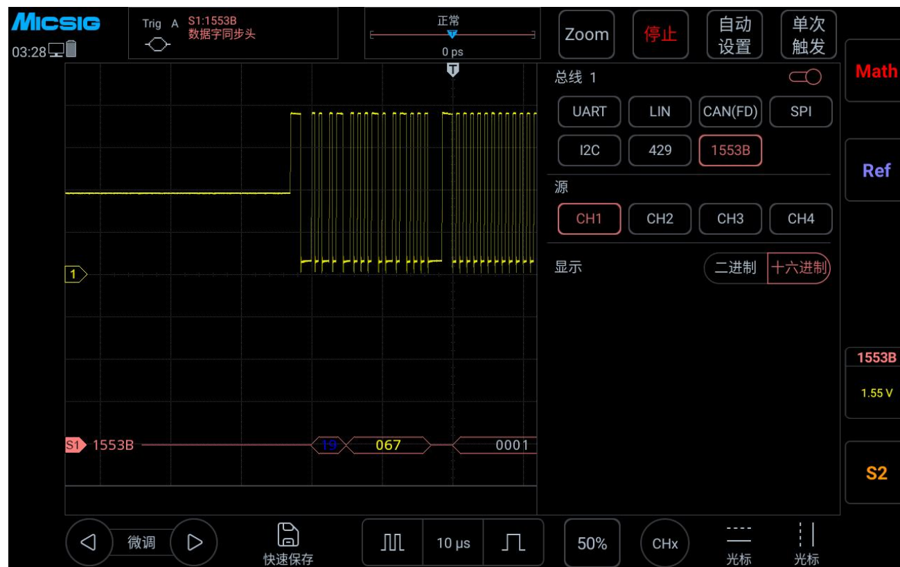
图 12-30 1553B 总线配置菜单
