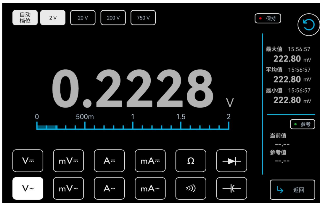
图 7-23 交流电压测量 V
