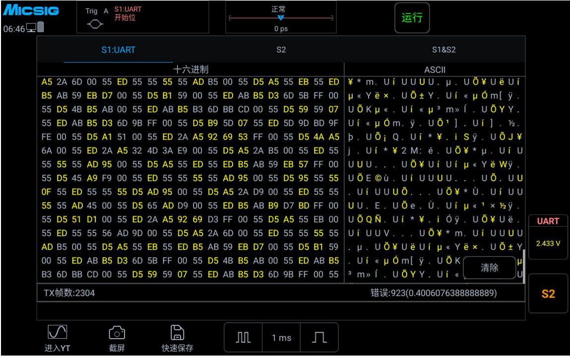
图 12-2 总线解码文本模式
