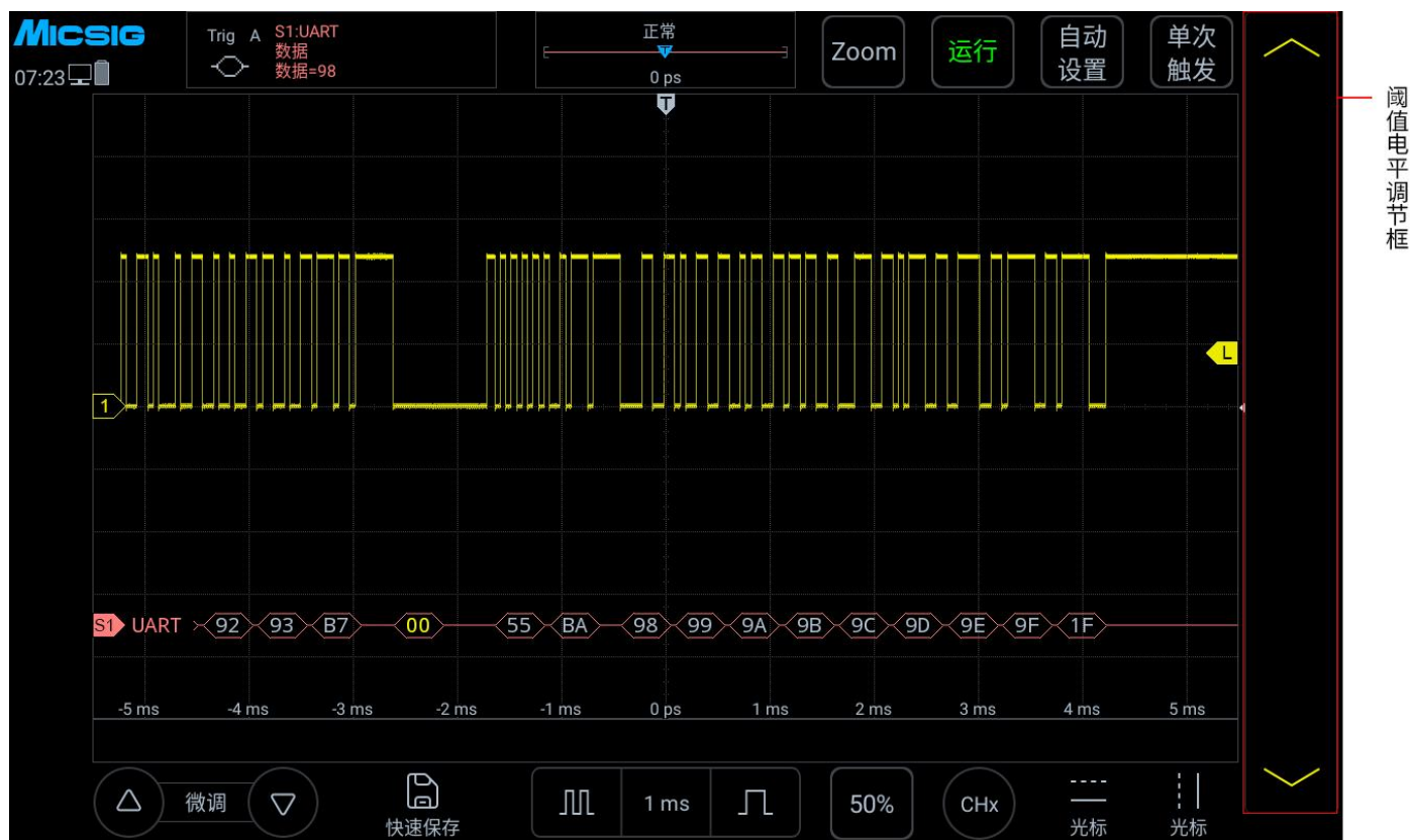
图 12-7 UART 解码电平调节
