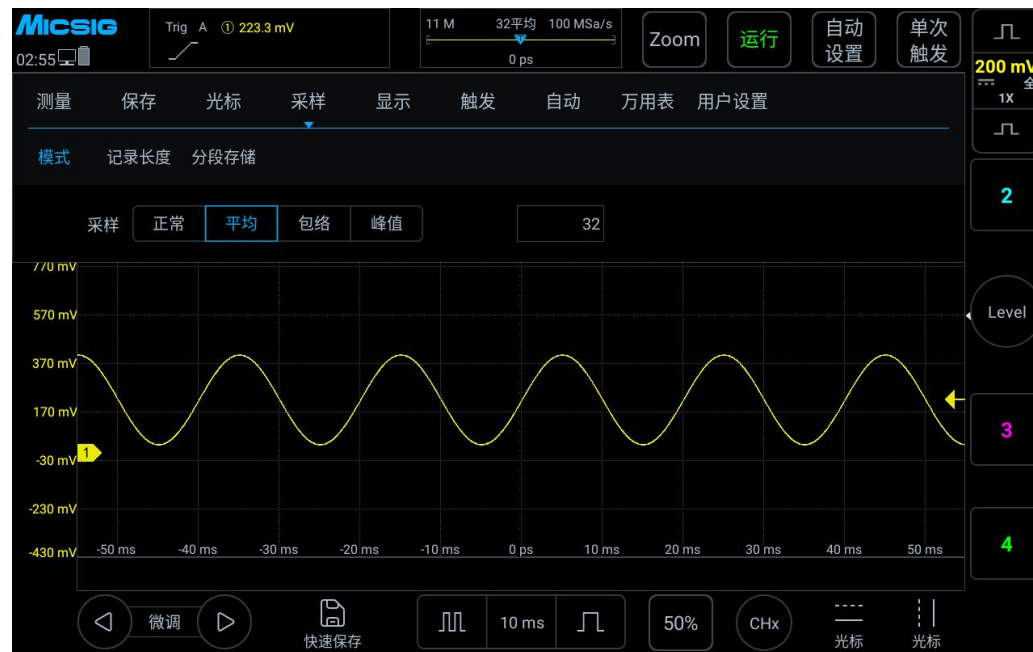
图 11-5 选择平均采样模式后的波形，平均数 32
