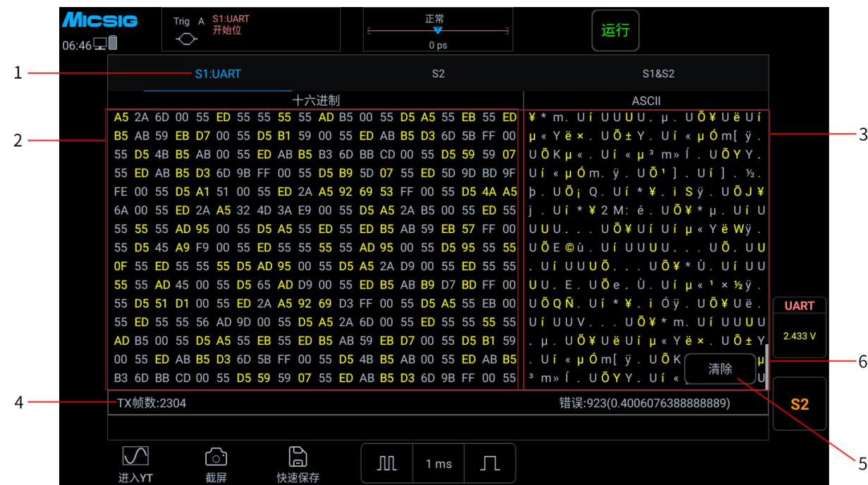
图 12-9 UART 文本界面
