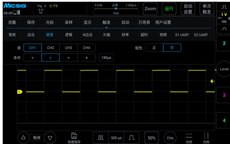
图 6-15 负极性脉冲电平翻转
