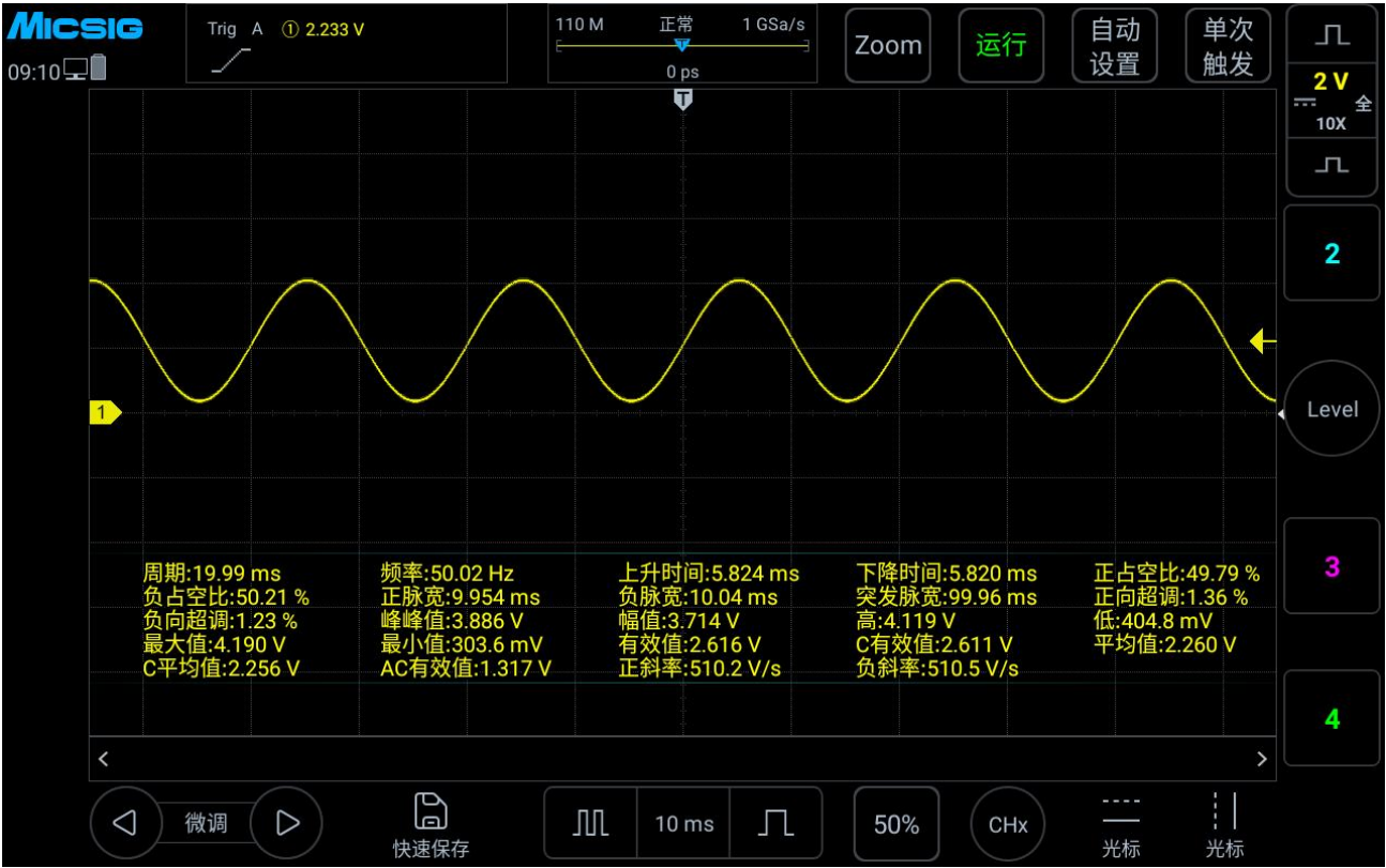
图 7-3 全部测量
