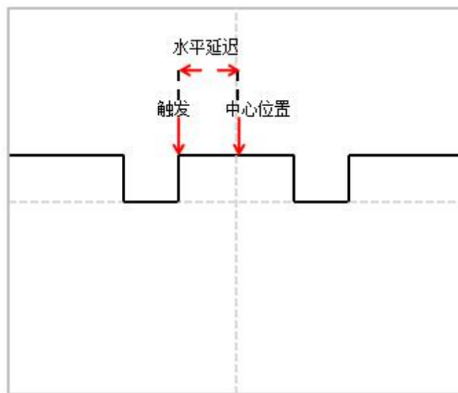
图 6-7 水平延迟
