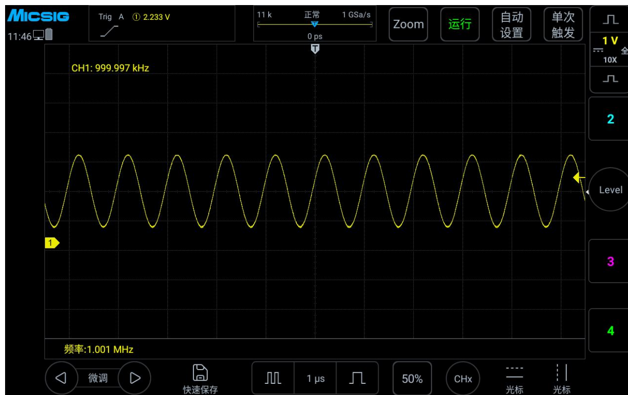
图 7-15 频率计测量
