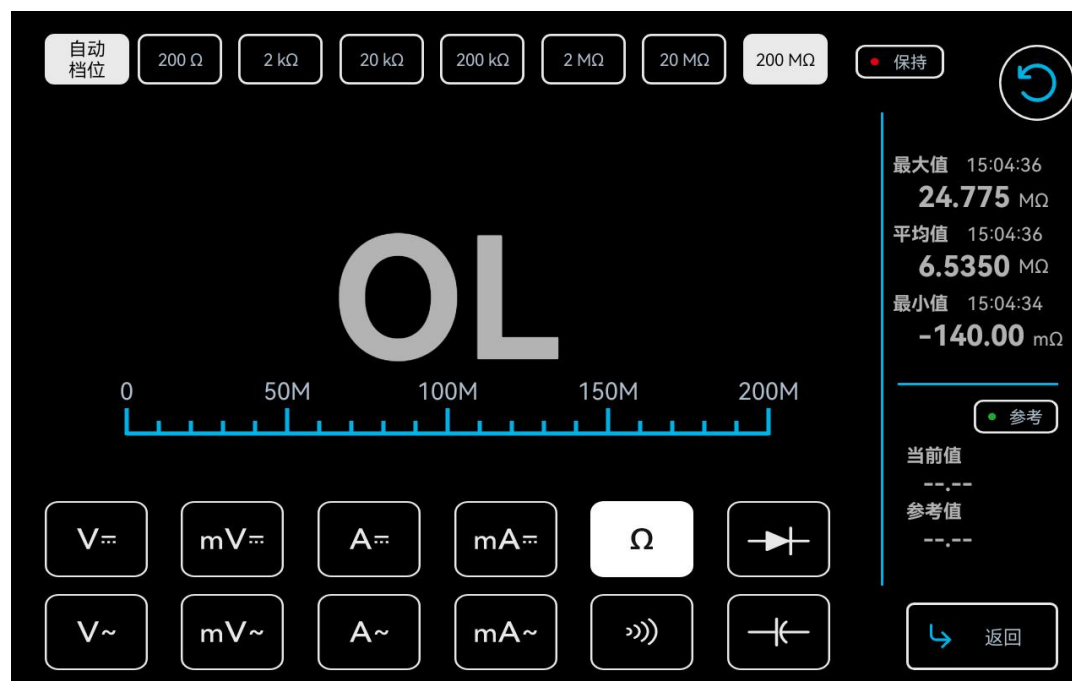
图 7-30 电阻测量
