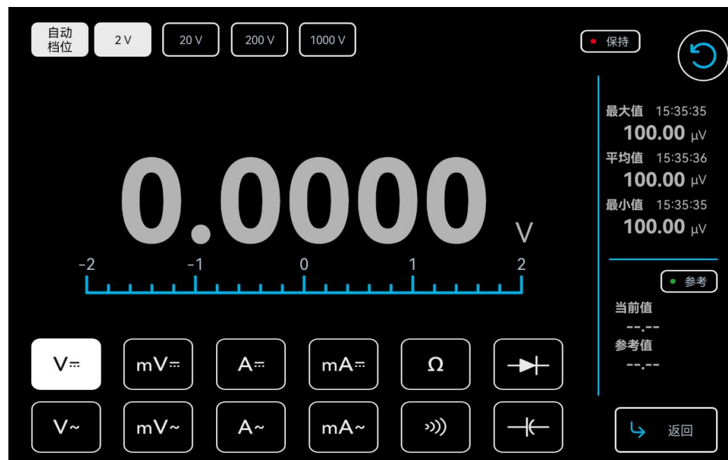
图 7-22 直流电压测量 V
