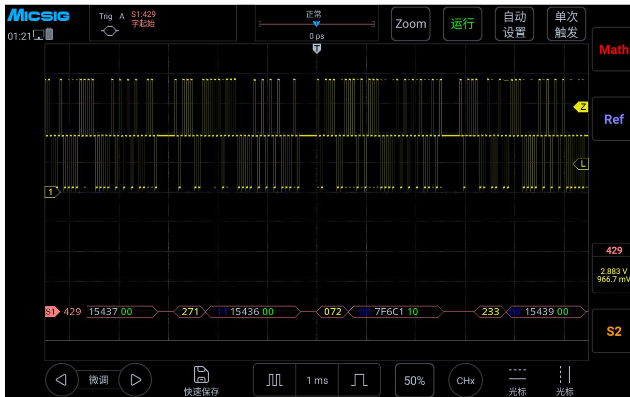
图 12-28 ARINC429 图形界面
