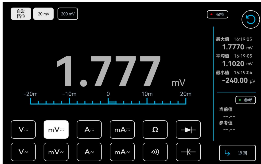
图 7-24 直流电压测量 mV
