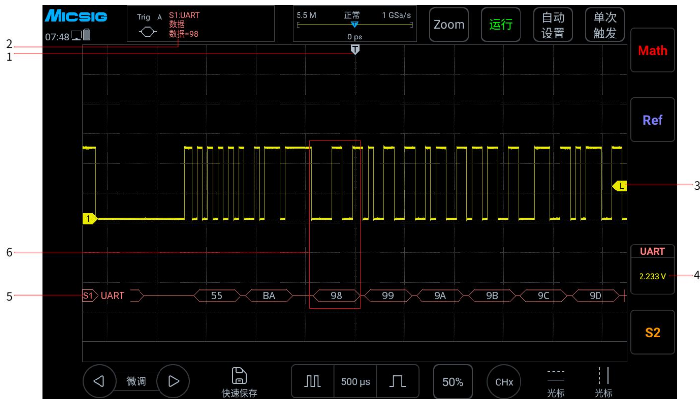
图 12-8 UART 图形界面
