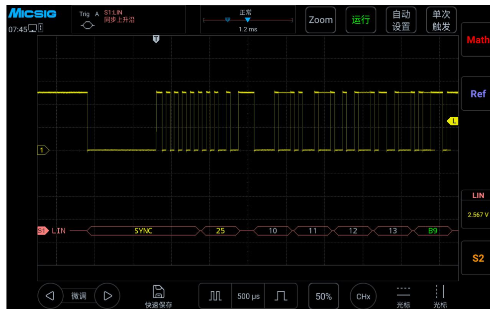
图 12-12 LIN 图形界面
