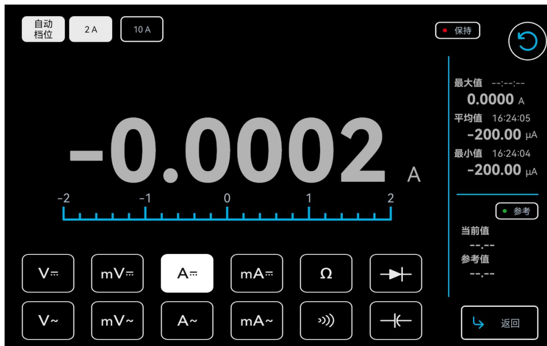
图 7-26 直流电流测量 A
