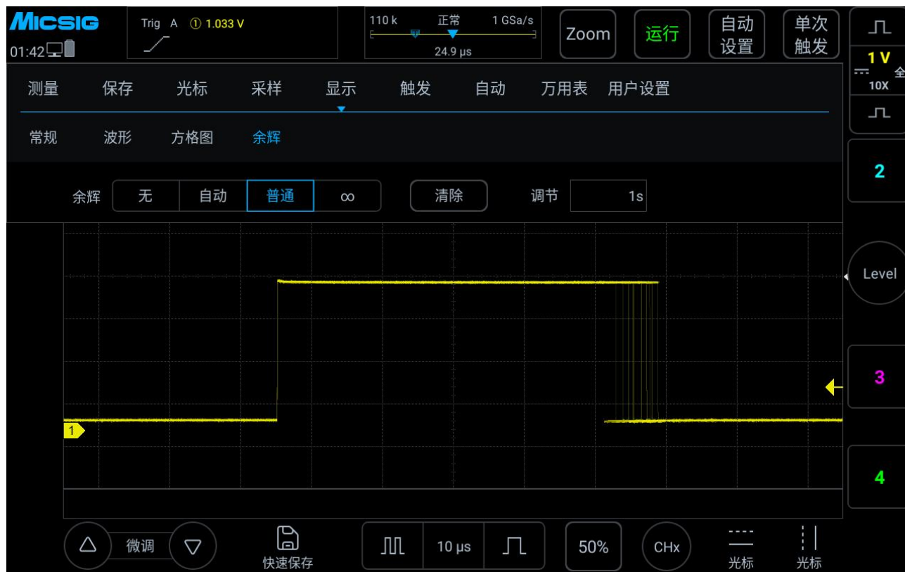
图 10-4 余辉时间调节
