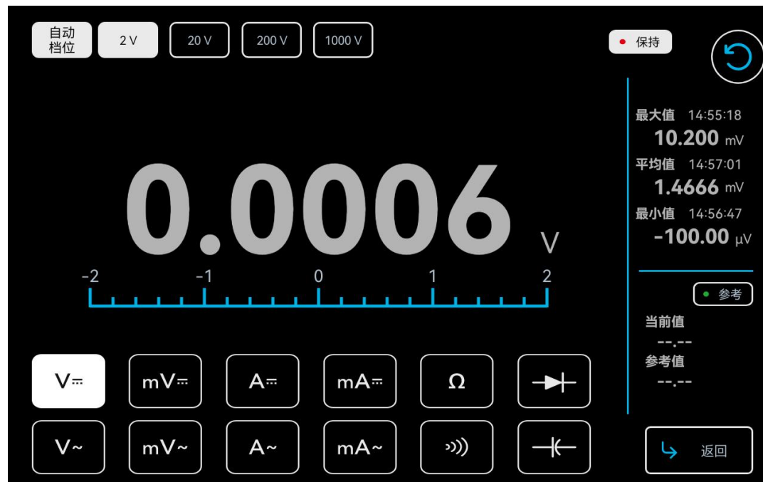
图 7-34 保持功能
