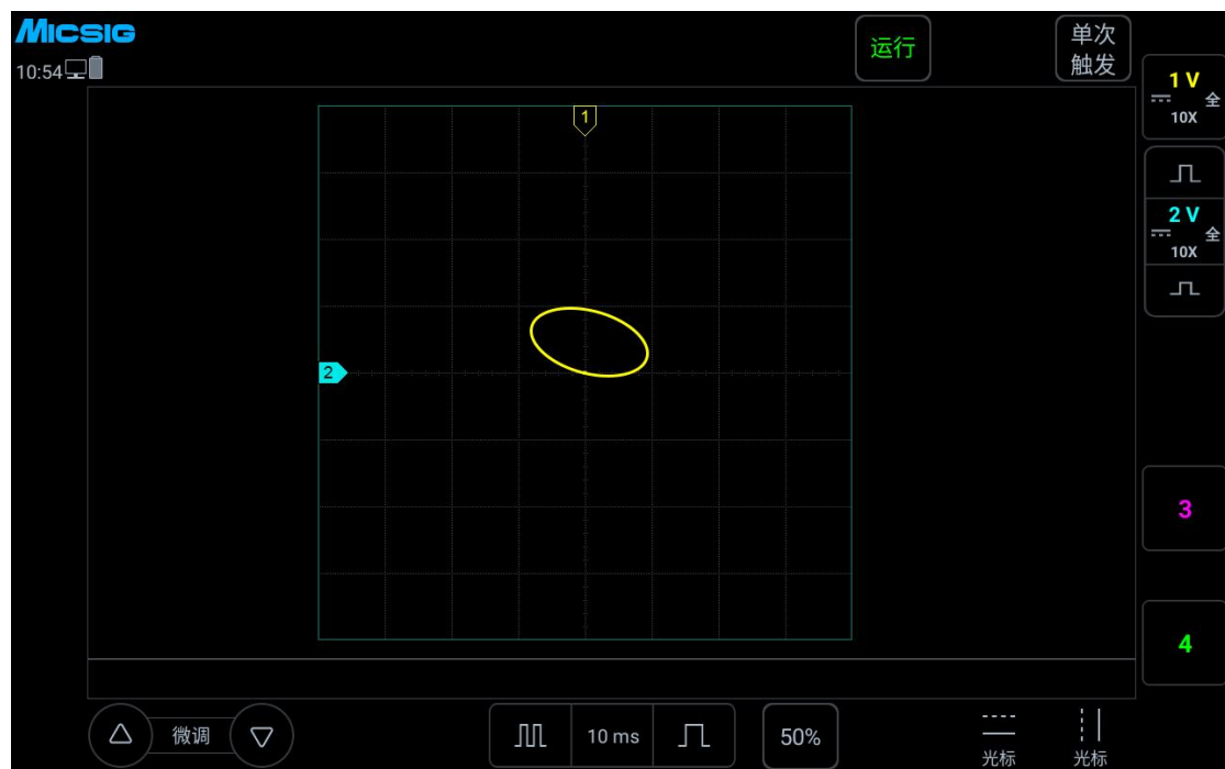
图 4-7XY 模式
