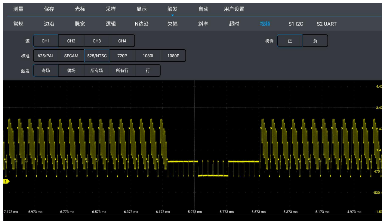
图 6-30 视频触发
