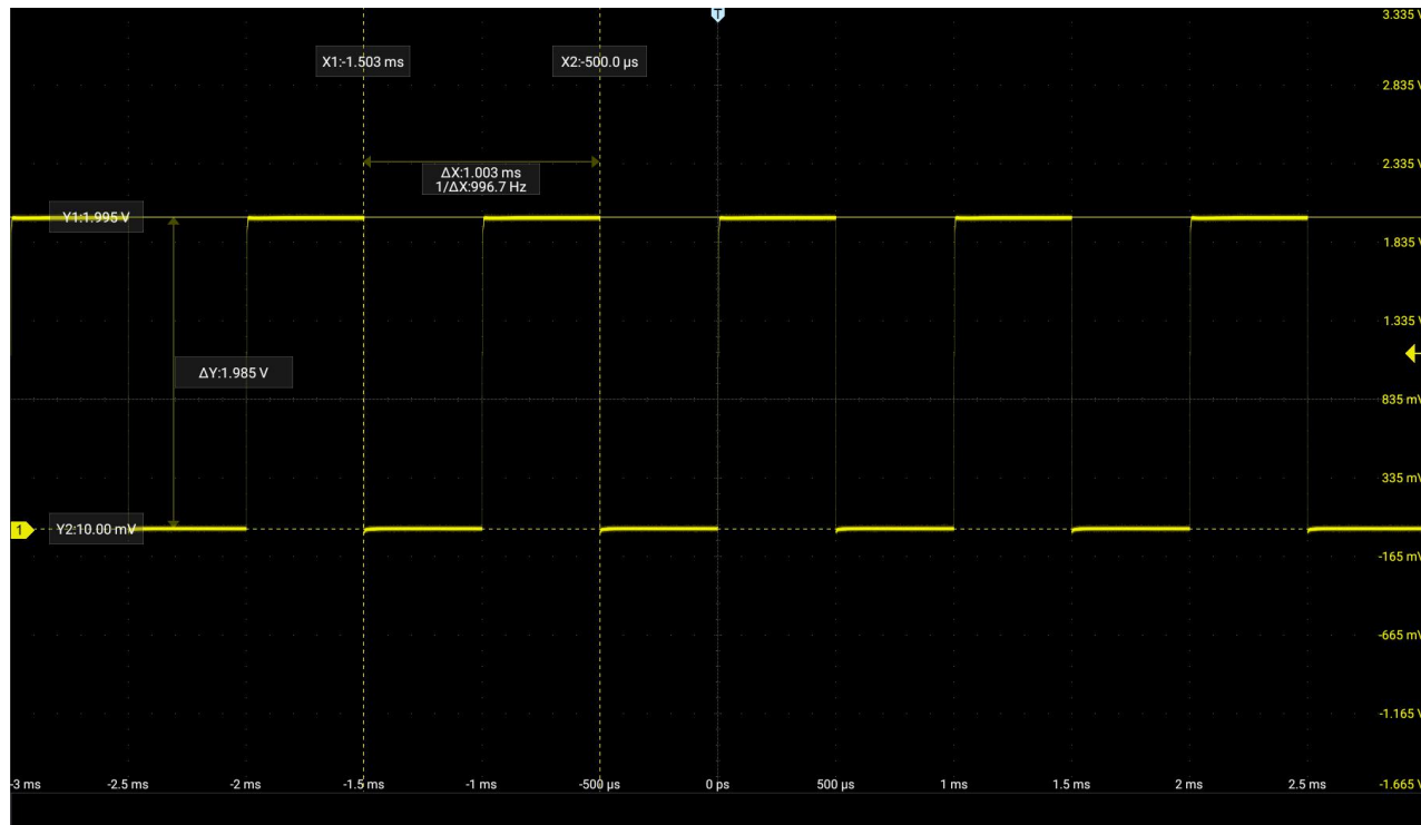
图 7-16 光标测量
