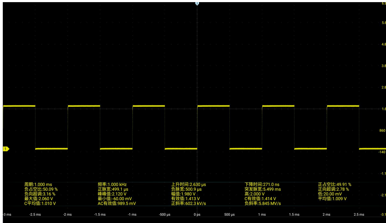
图 6-3 全部测量
