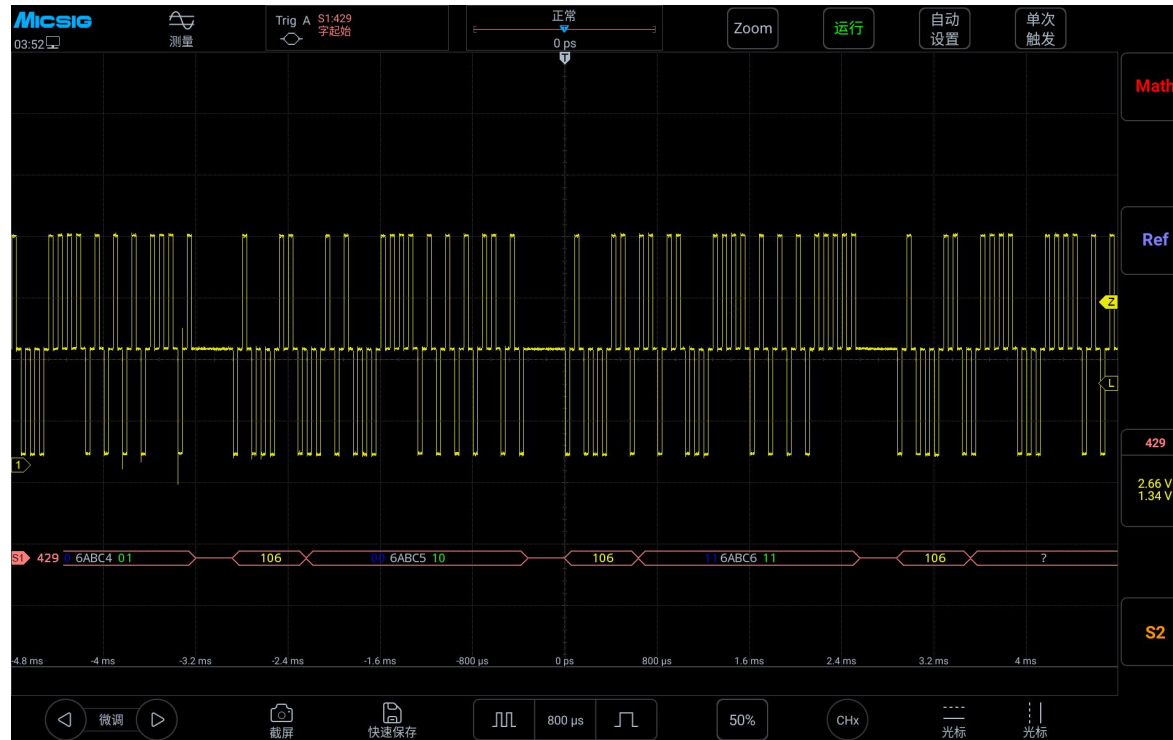
图 11-28 ARINC429 总线解码结果
