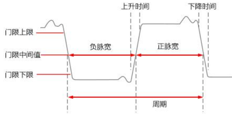
图 6-4 时间参数
