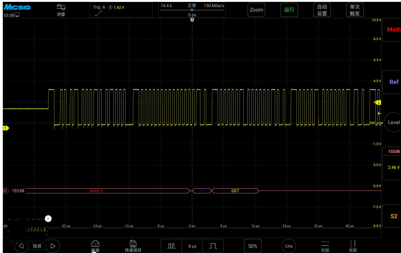
图 11-32 1553B 总线解码结果
