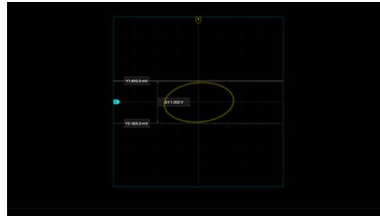
图 6-19 XY 模式中，光标测量
