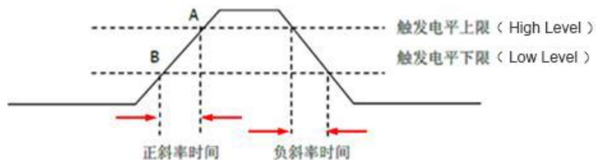
图 5-26 正斜率时间/负斜率时间
