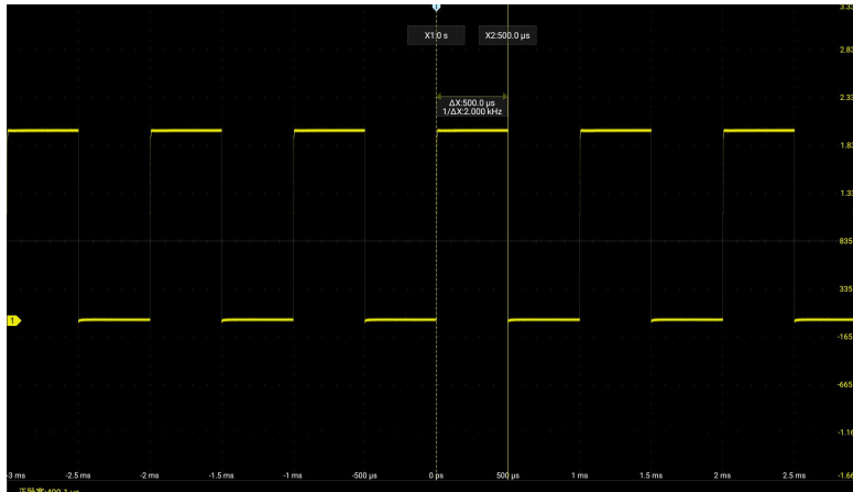
图 6-18 光标测量脉冲宽度
