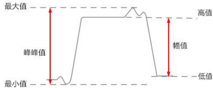
图 6-7 电压测量
