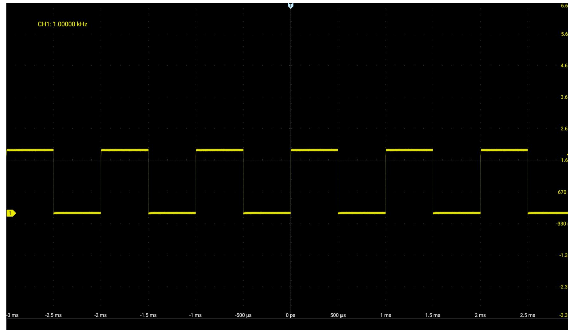
图 6-15 频率计测量
