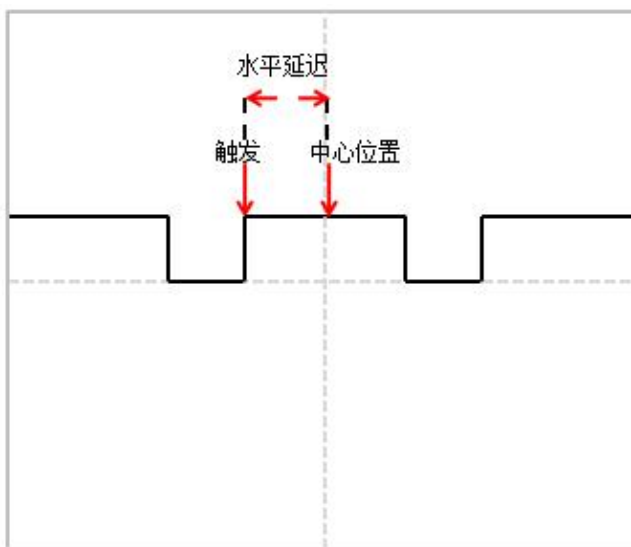
图 5-7 水平延迟
