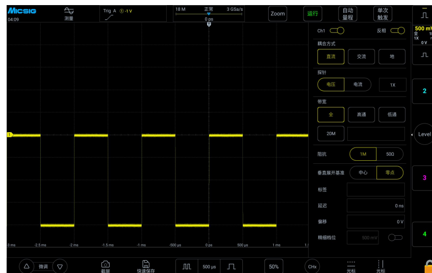
图4-15 反相后
