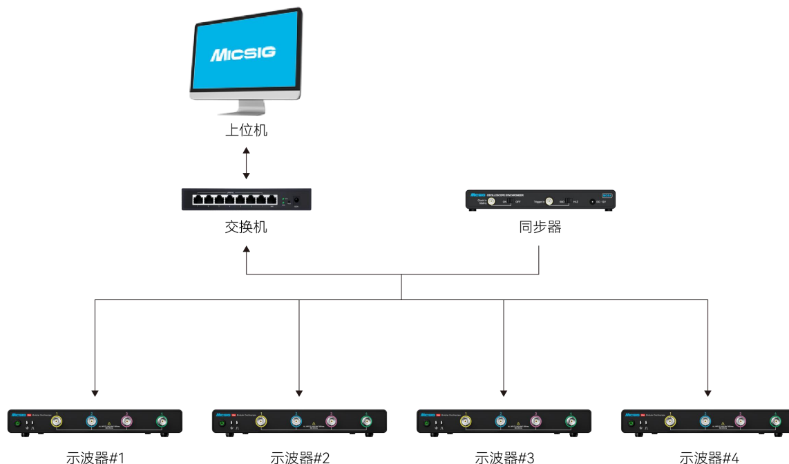
图 2-4 示波器矩阵式连接
