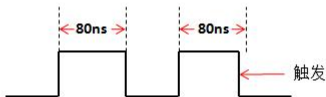
图 5-19 触发时间 T \neq 80\text{ns}
