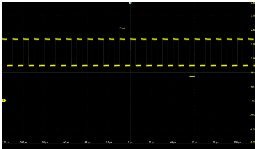
图 5-3 周期信号中有异常信号
