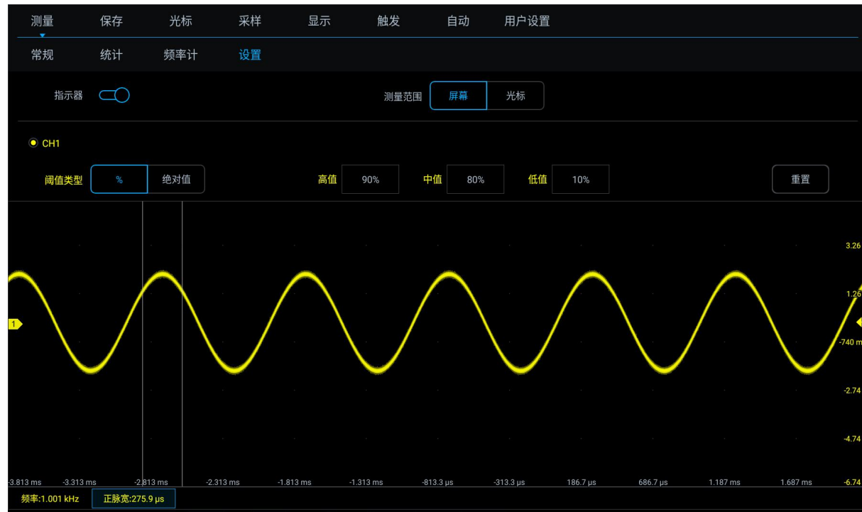
图 6-13 阈值中值设为 80%时的脉宽
