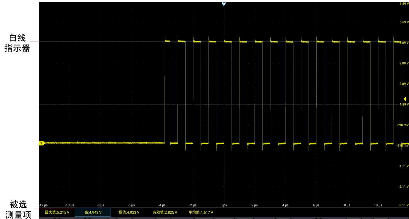
图 6-11 指示器
