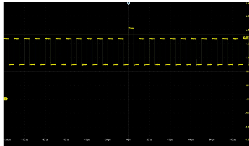
图 5-4 通过设置触发电平捕获到该异常信号
