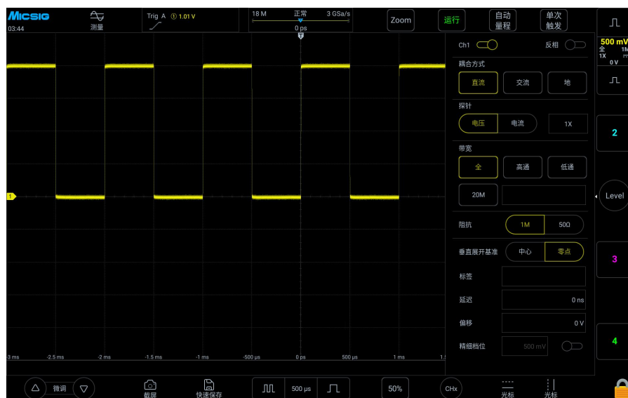
图4-7 DC耦合
