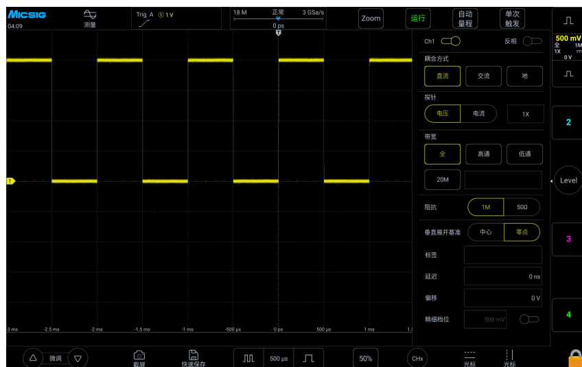
图4-14 反相前
