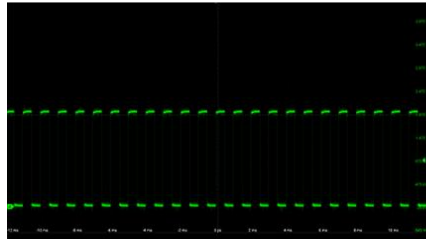
图 10-6 带毛刺的波形，正常采样模式
