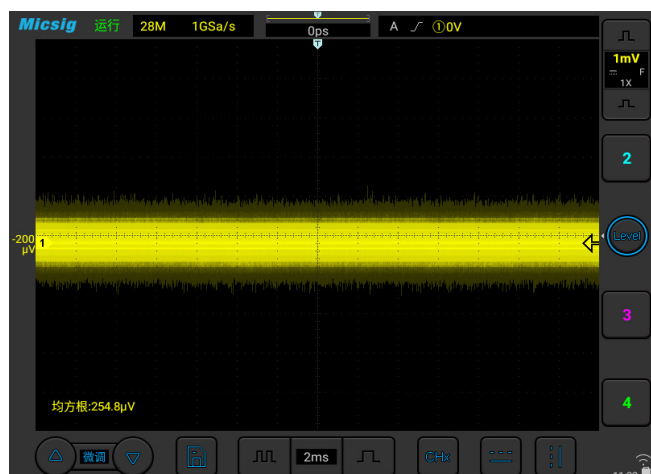
全带宽下底噪 254.8μVrms
