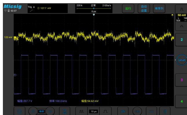
CH1: 在 100kHz, 207.7V 信号下输出的共模信号幅度 94.62mV, 共模抑制比 >-60dB
